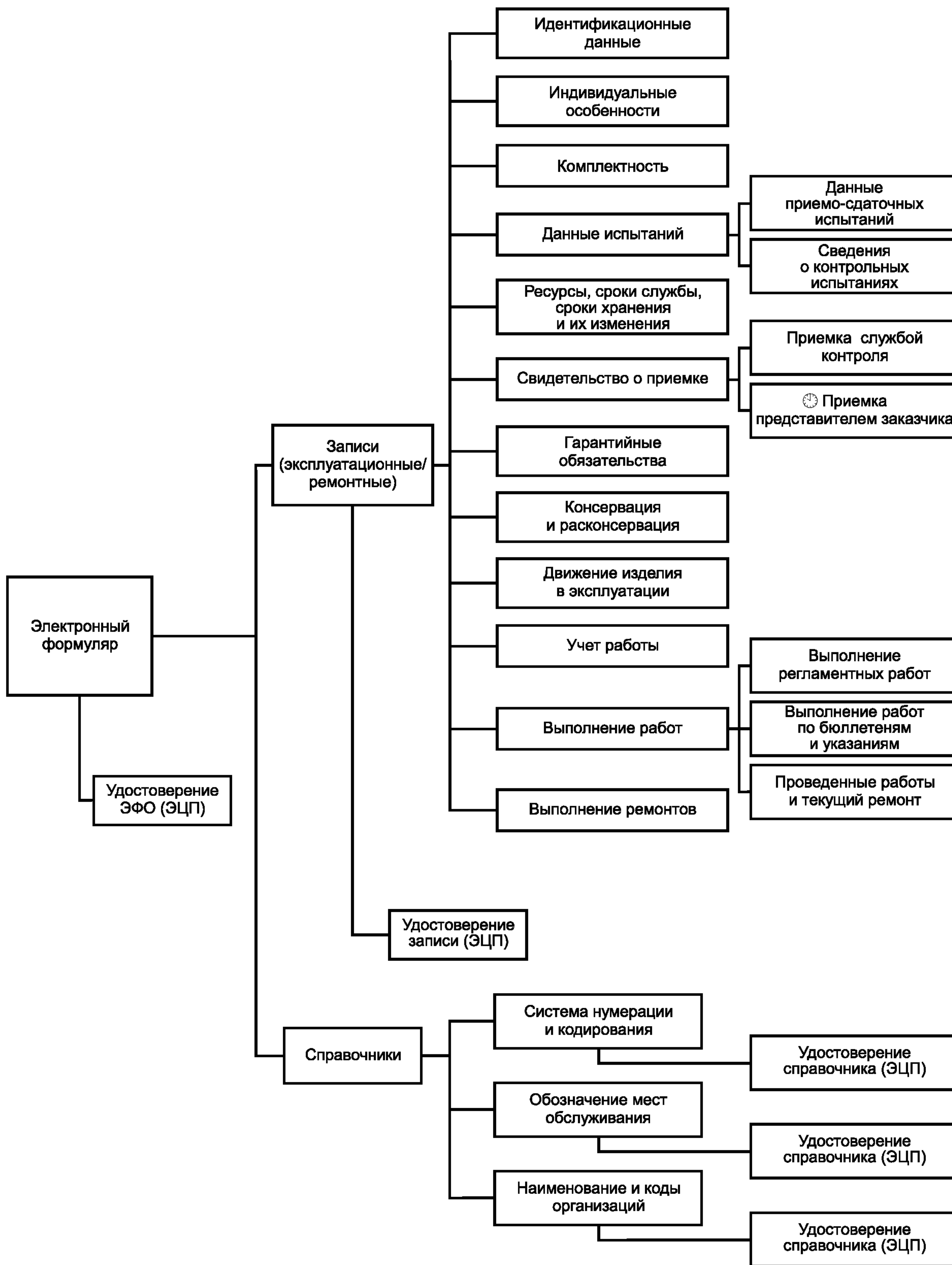
Рисунок Б.1 — Логическая структура электронного формуляра
