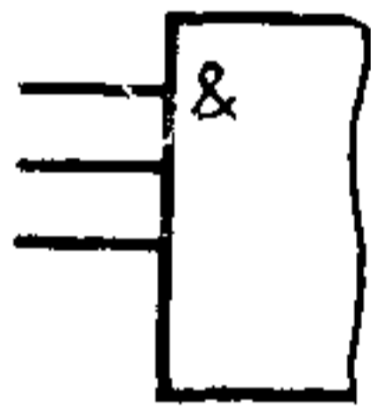
а — группа выводов объединена по И,
