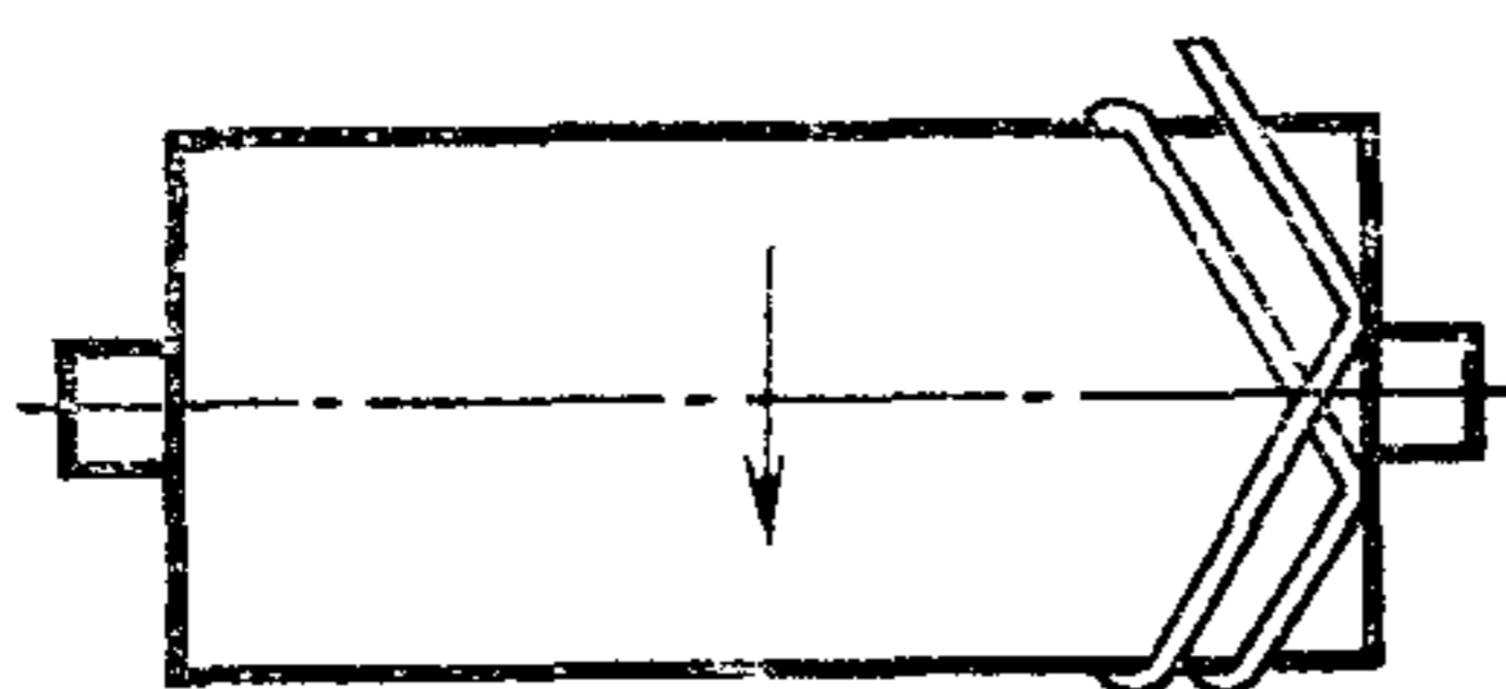
Отстающая намотка
