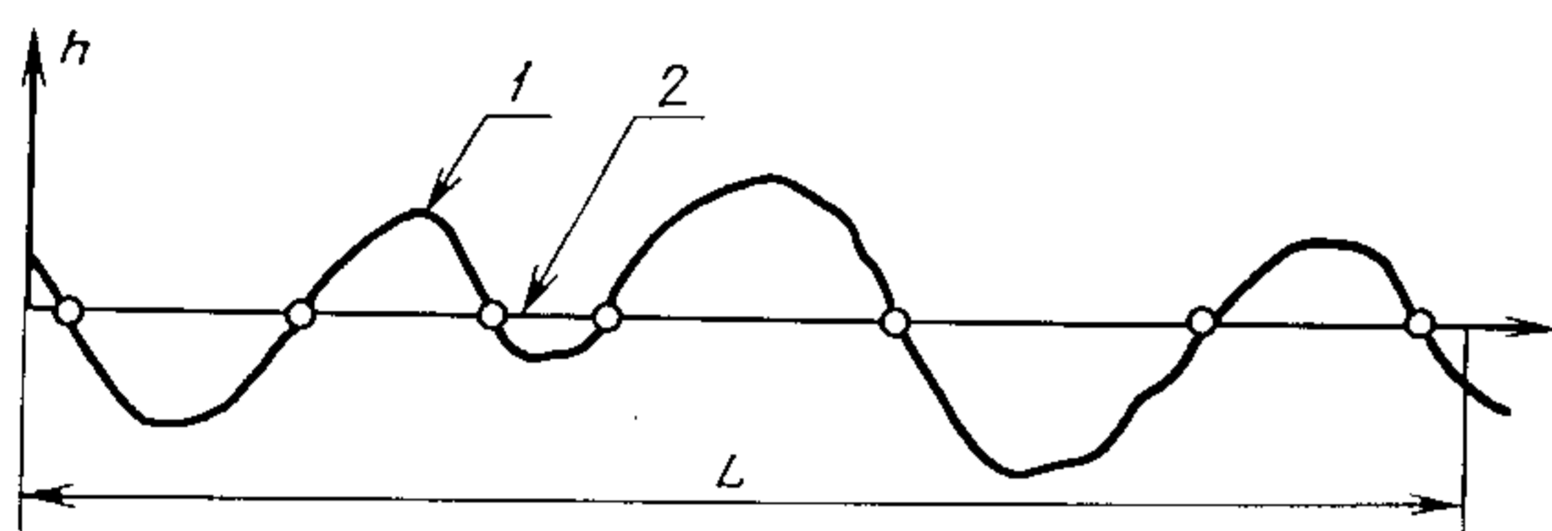
1 — реальный профиль; 2 — средняя прямая
