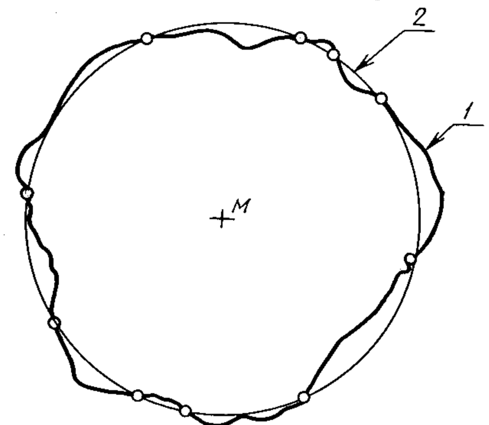
1 — реальный профиль; 2 — средняя окружность
