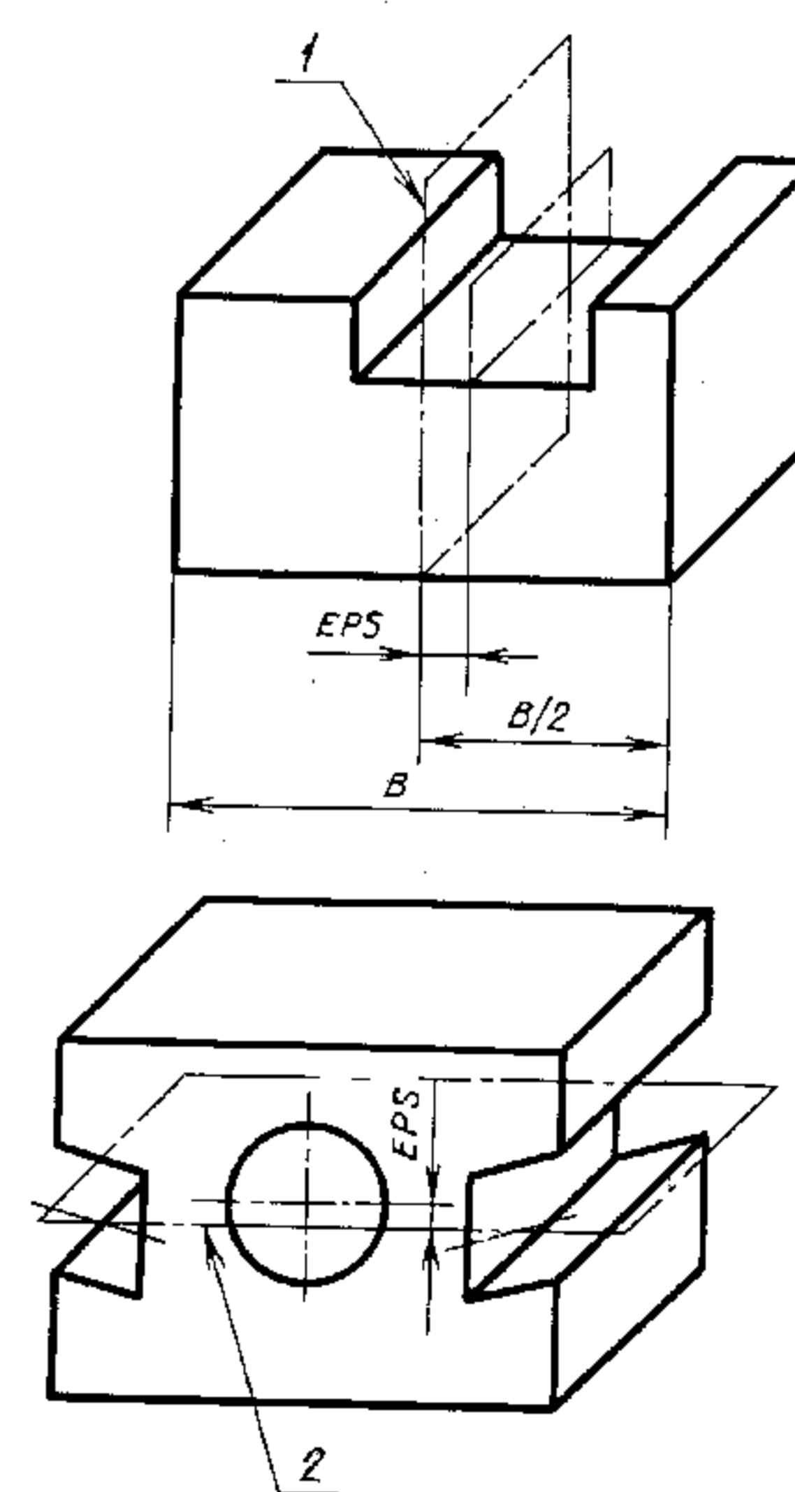
1 — база (плоскость симметрии базового элемента); 2 — база (общая плоскость симметрии)
