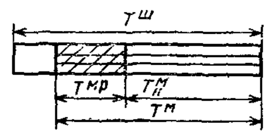
Черт. 2. Хронограммы штучного времени
