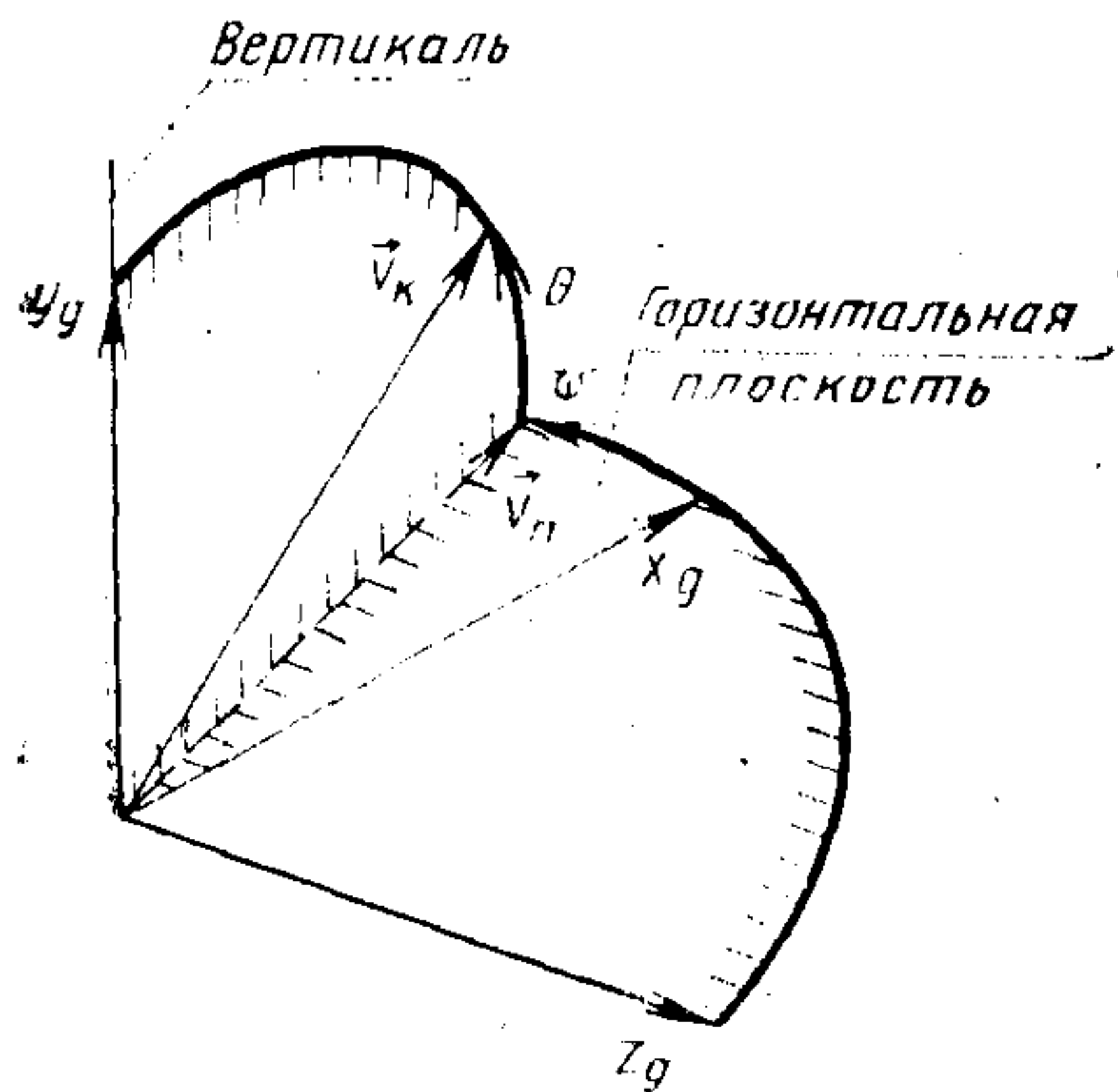
Черт. 4
