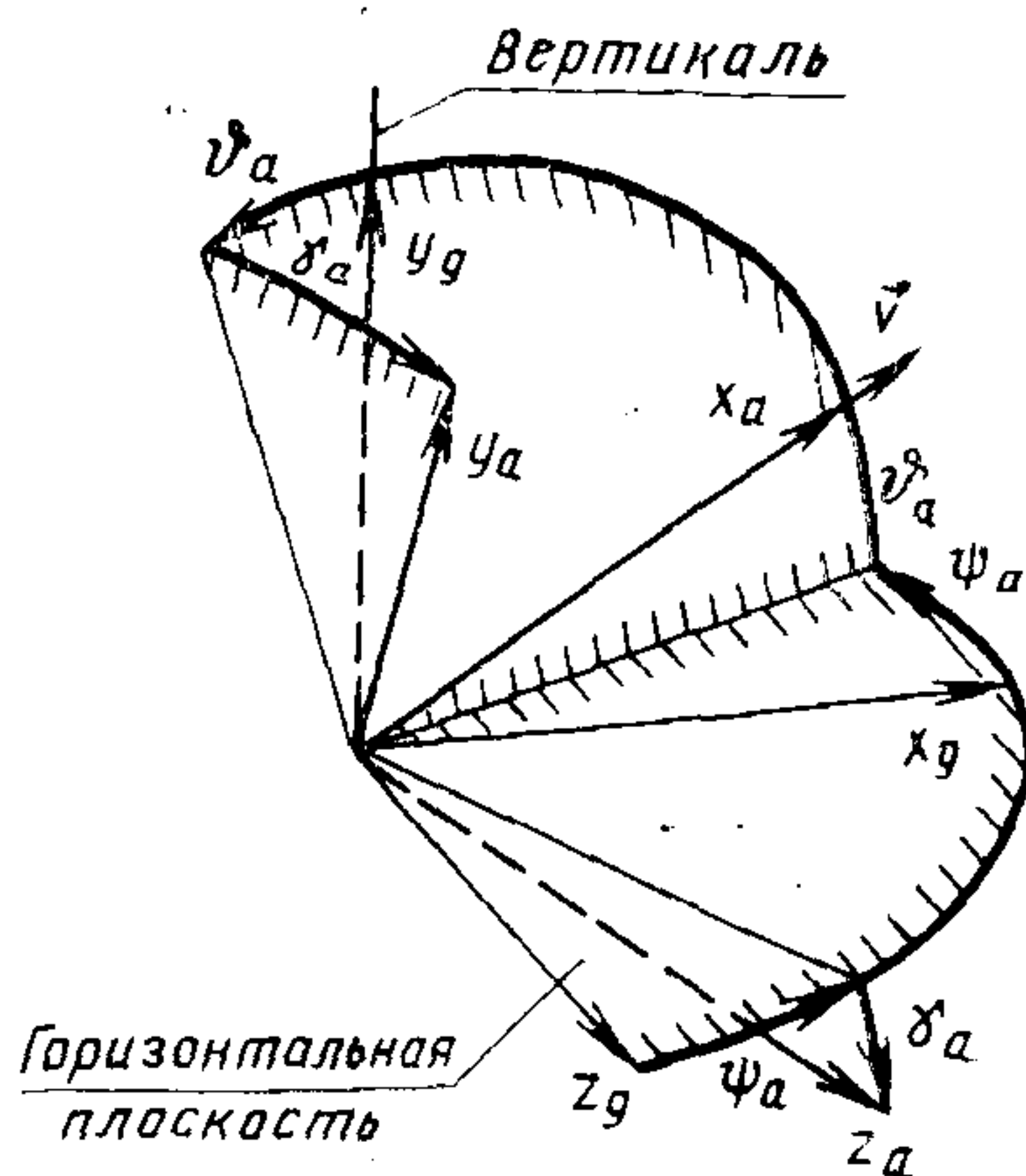
Черт. 3
