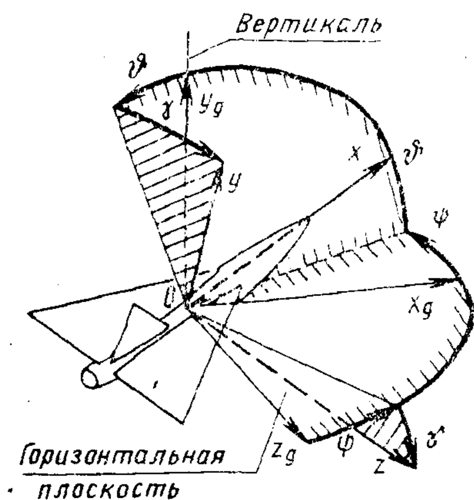
Черт. 2
