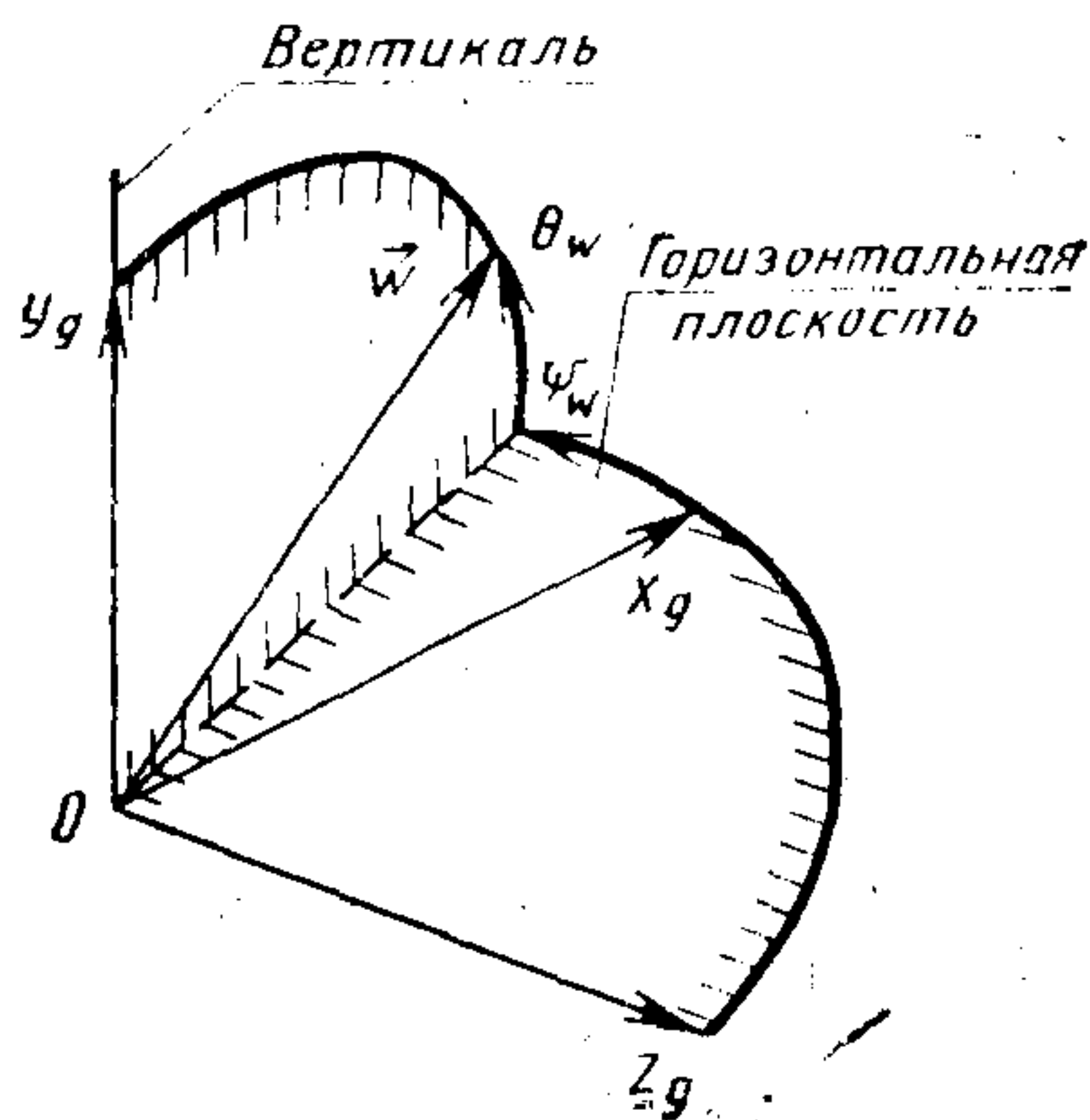
Черт. 5
