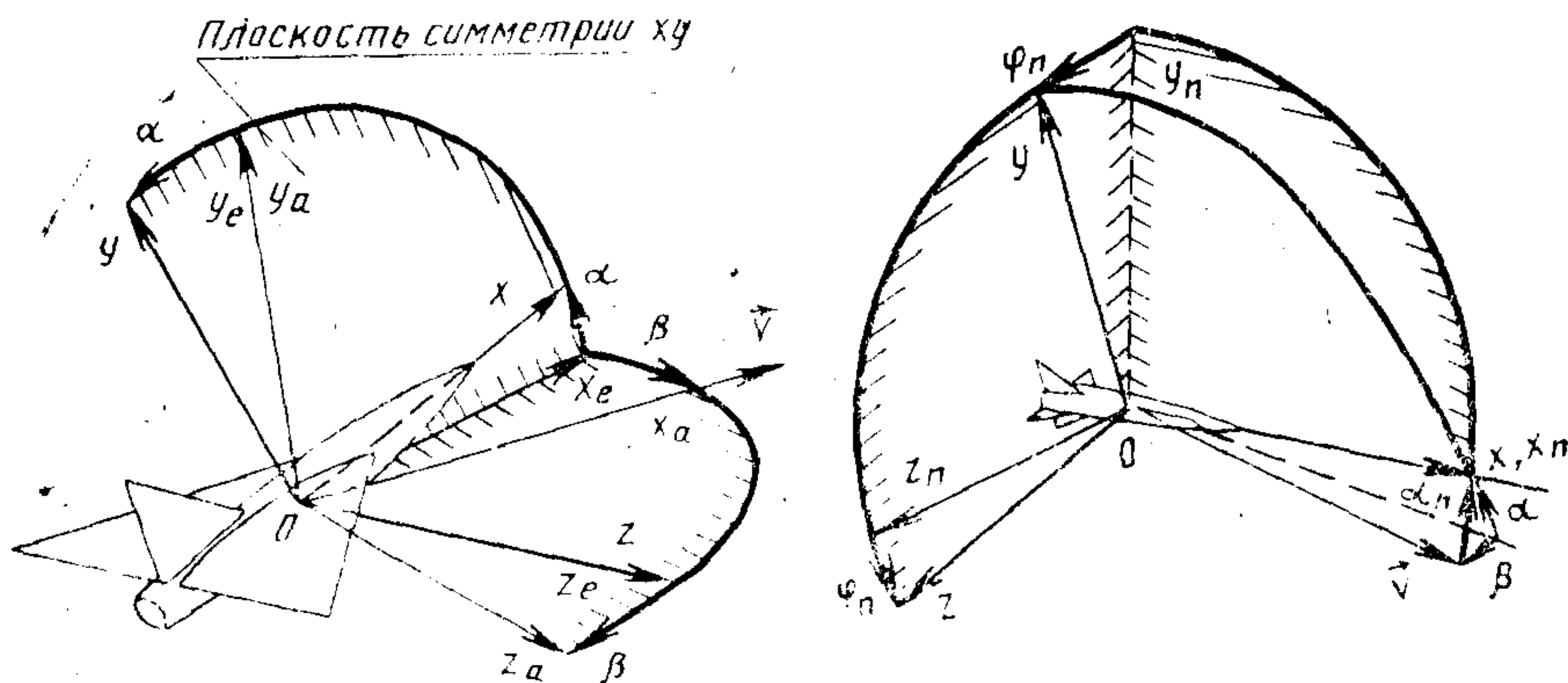
Черт. 1
