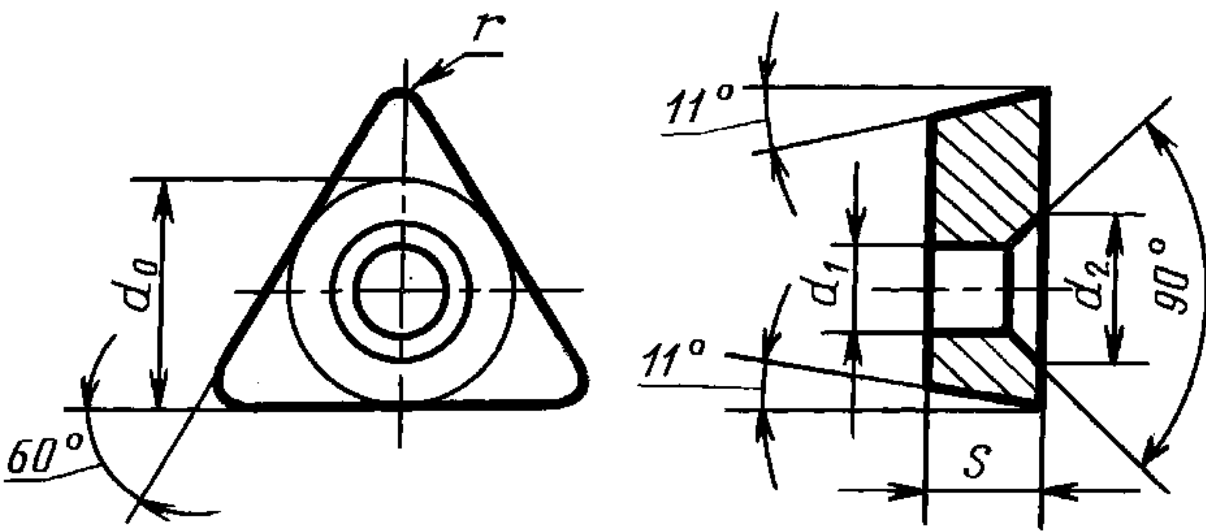
Размеры, мм
