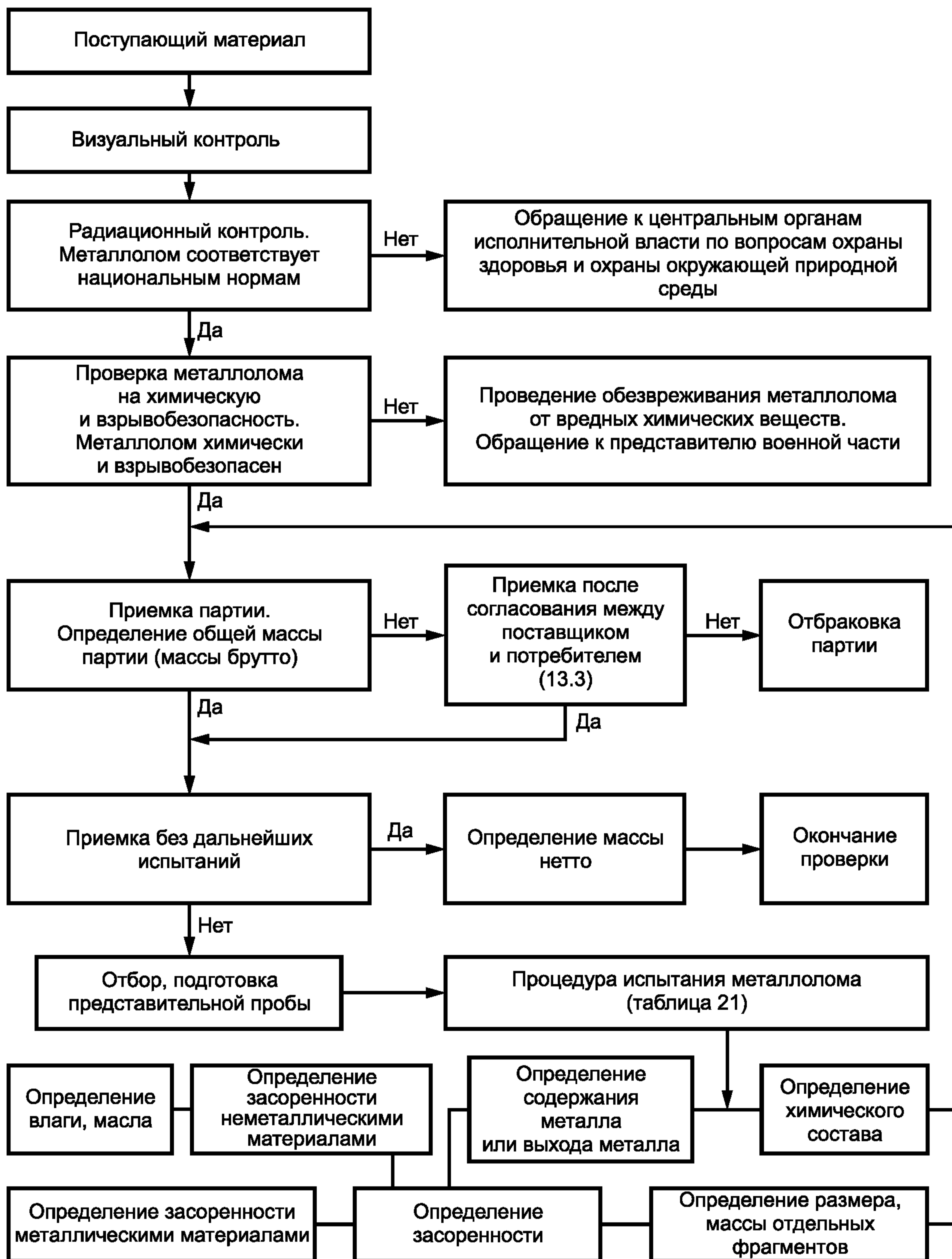
Рисунок 1 — Схема проверки поступающего металлолома
