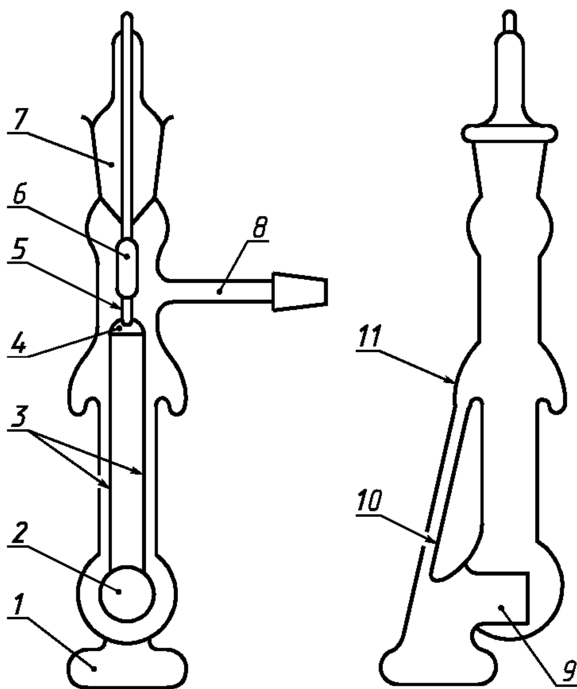
Общий вид тензиометра
