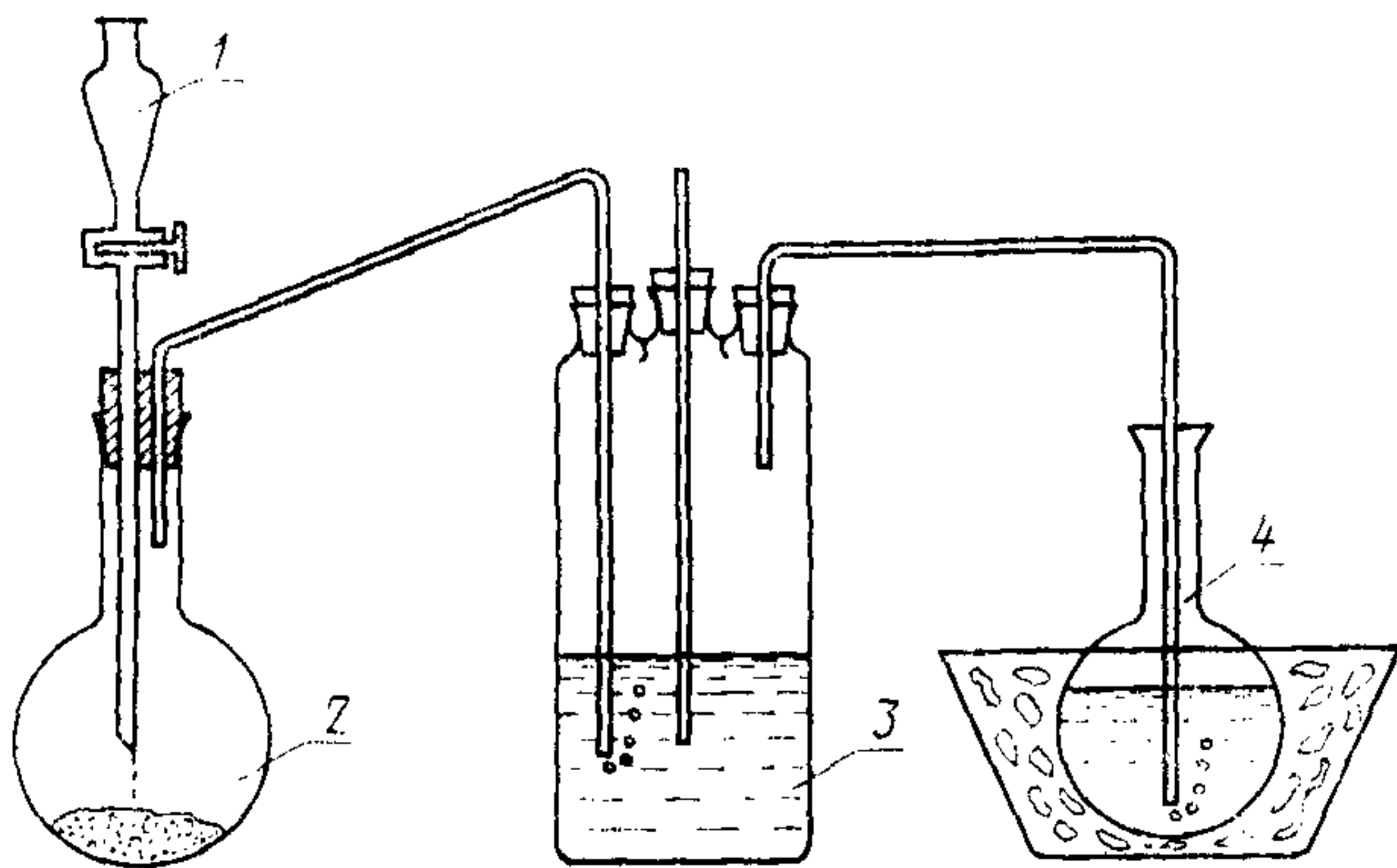
Прибор для получения хлора
