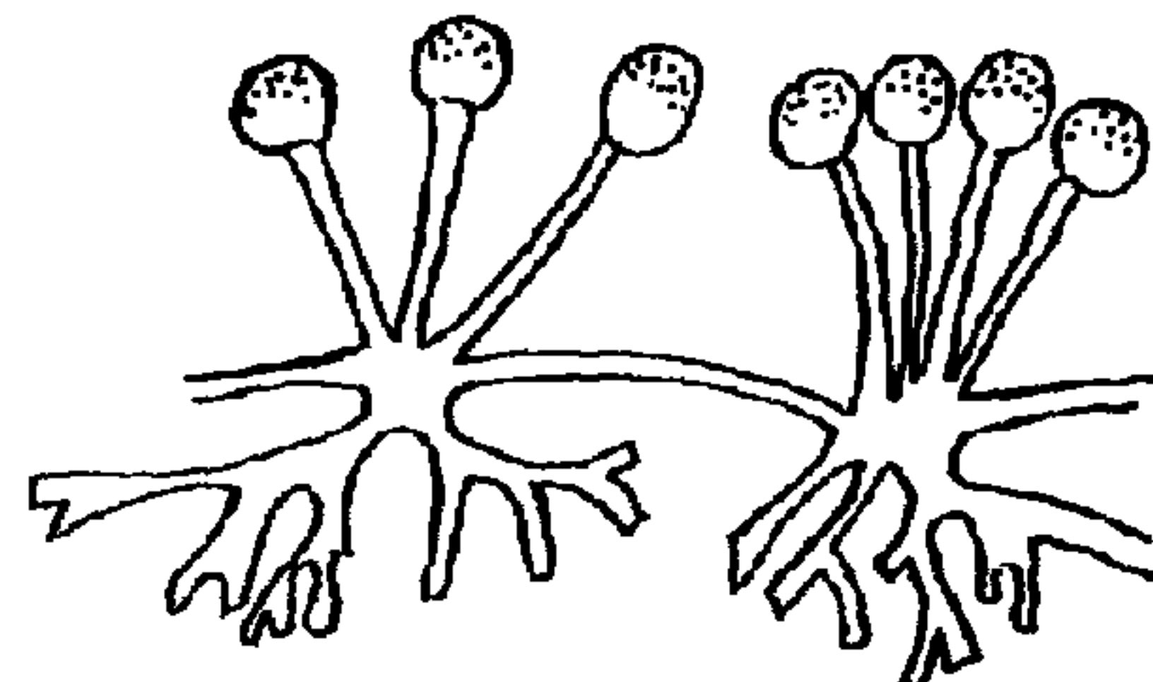
Рисунок В.2 — Ризопус ( Rhizopus Ehrent)
