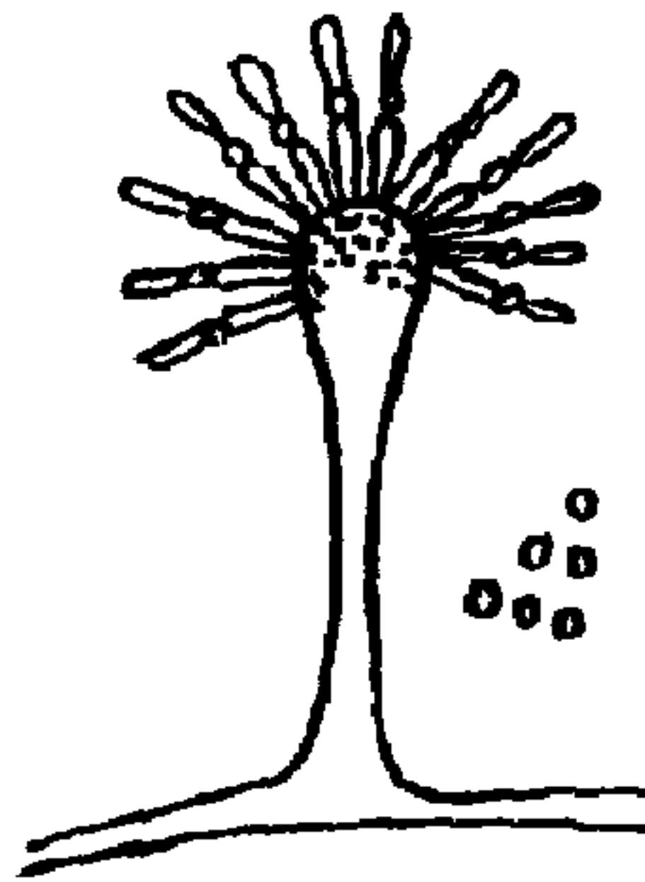
Рисунок В.5 — Аспергиллус (Aspergillus Mich)
