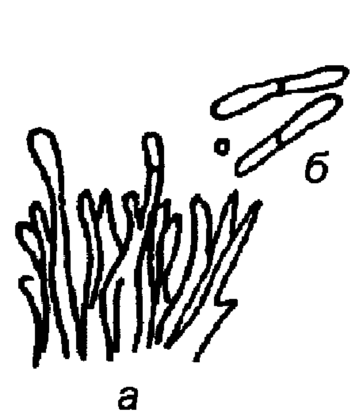
а — пучок конидиеносцев с конидиями б — конидии (увеличено)
