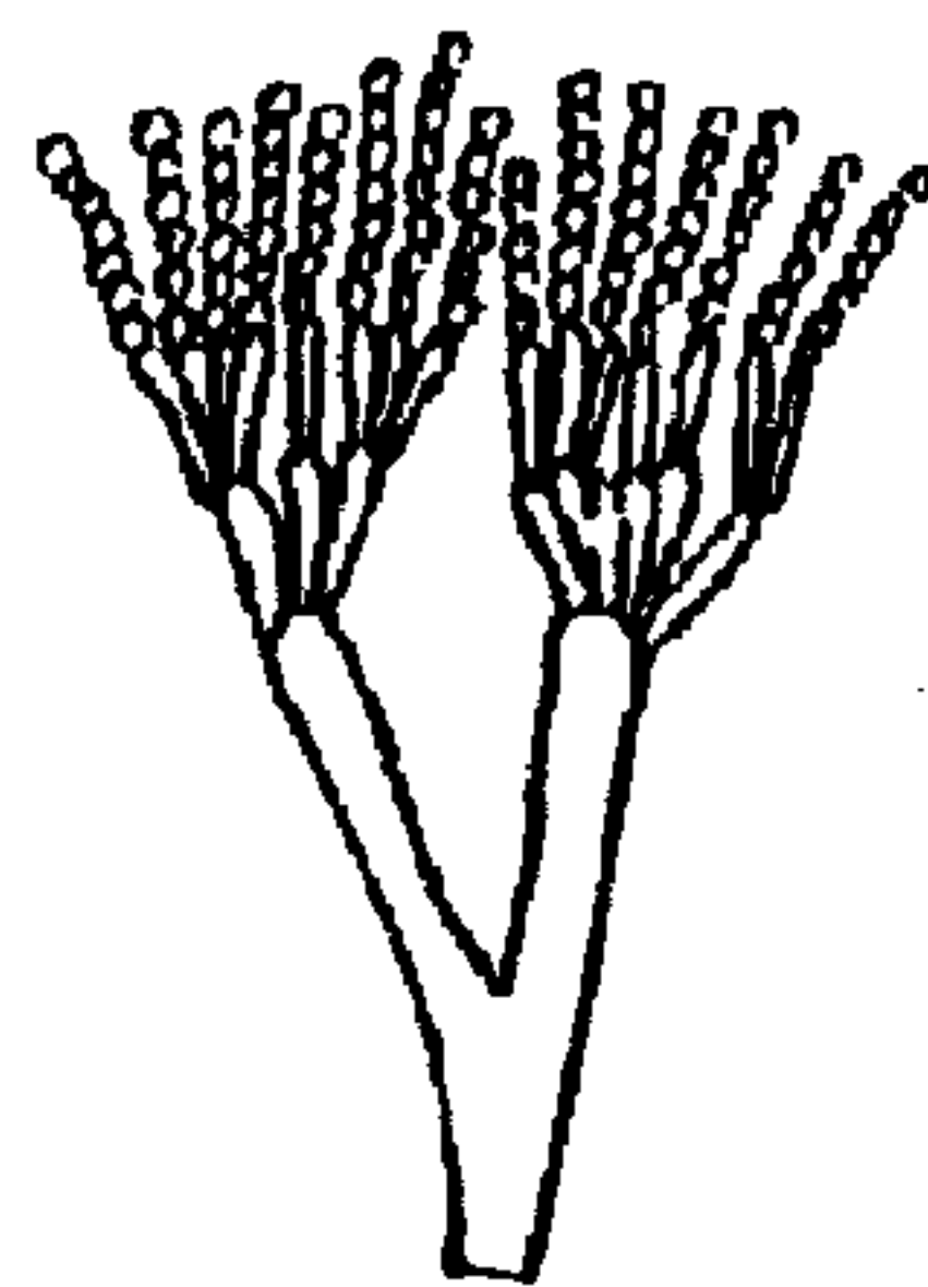
Рисунок В.1 — Пеницил- лиум ( Penicillium Link)
