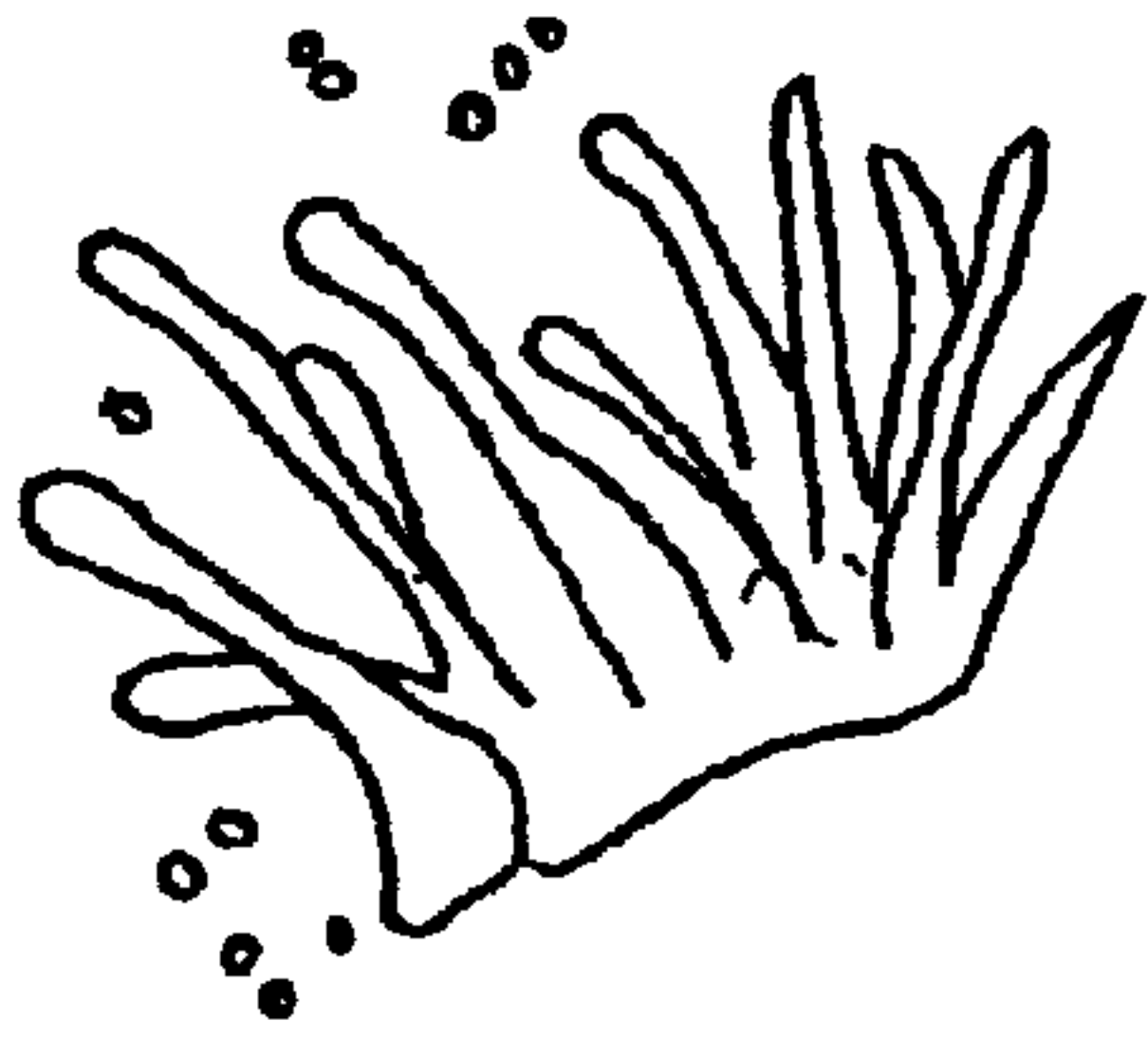
Рисунок В.4 — Кладоспориум (Cladosporium Link)
