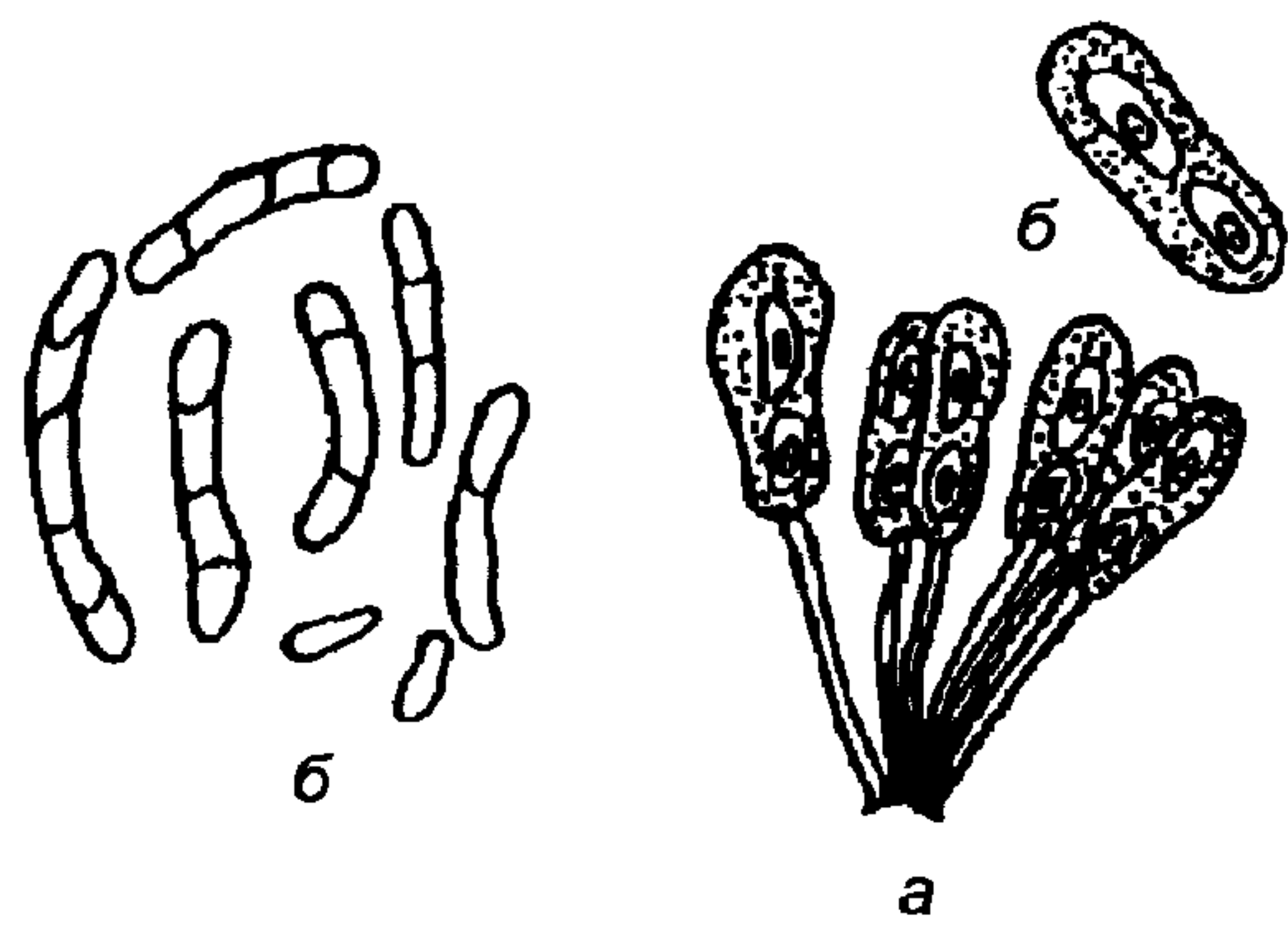
а — телейтоспоры б — телейтоспора (увеличено)
