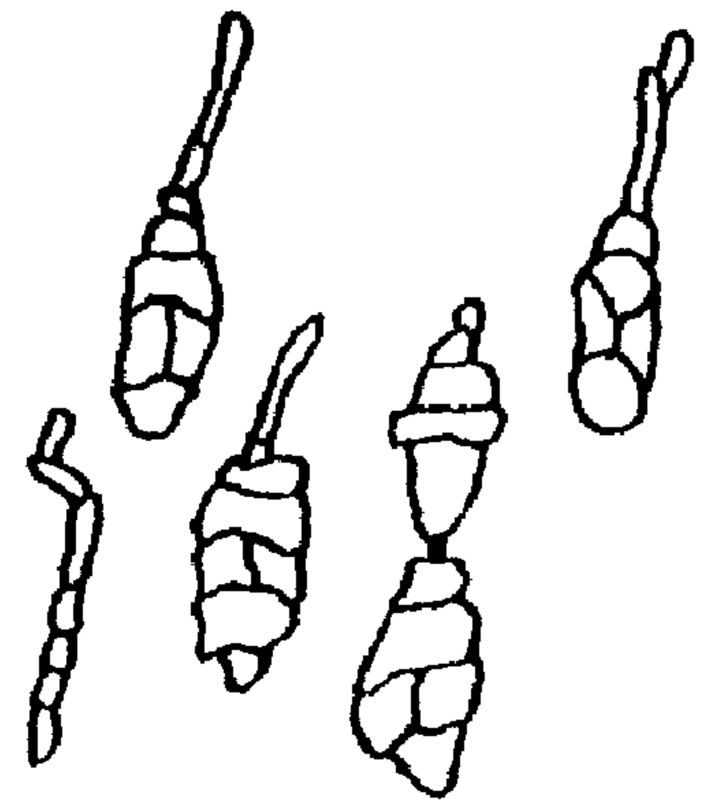
Рисунок В.6 — Альтернария (Alternaria Ness)
