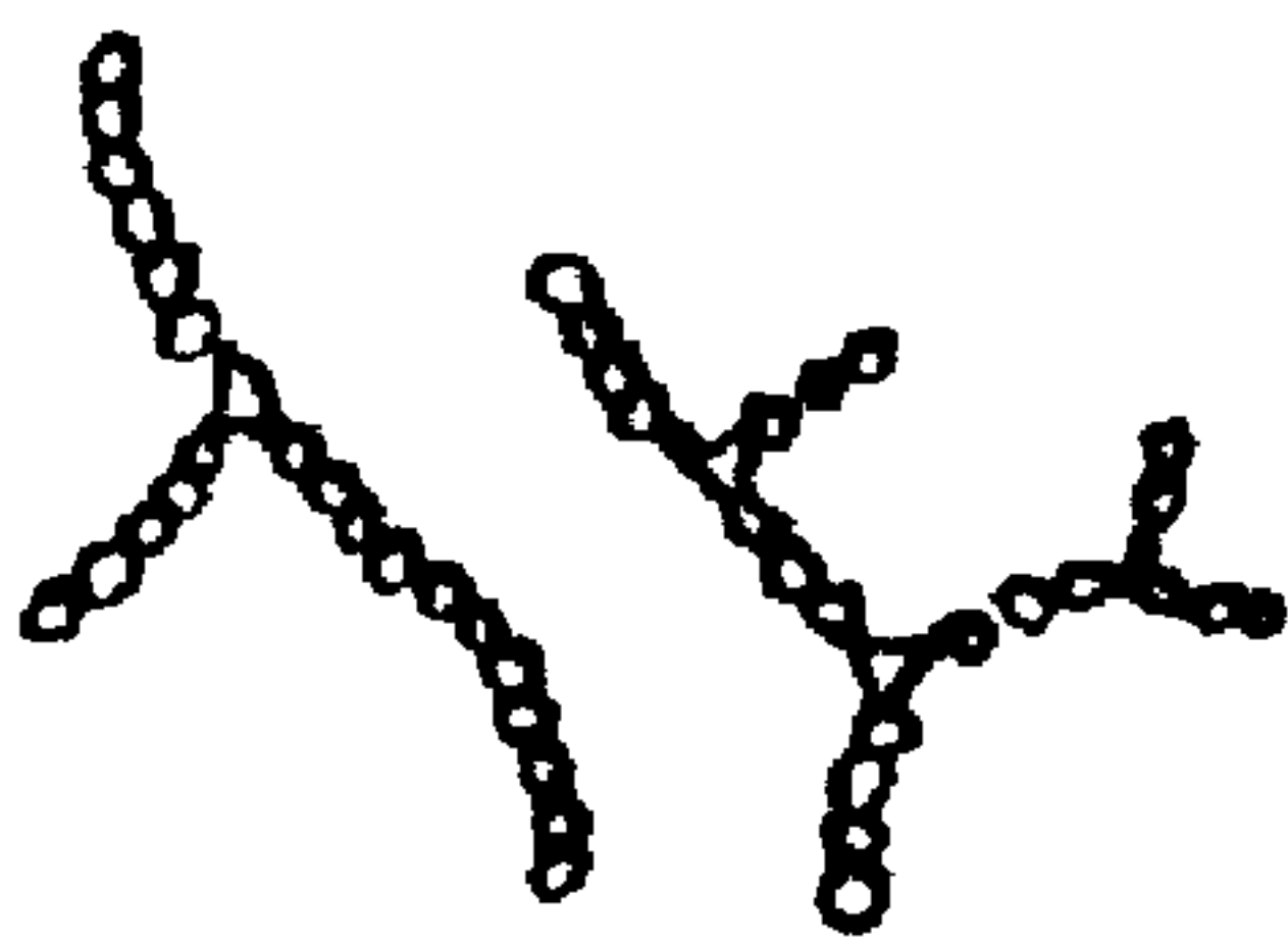
Рисунок В.7 — Монилия (Monilia Pers)
