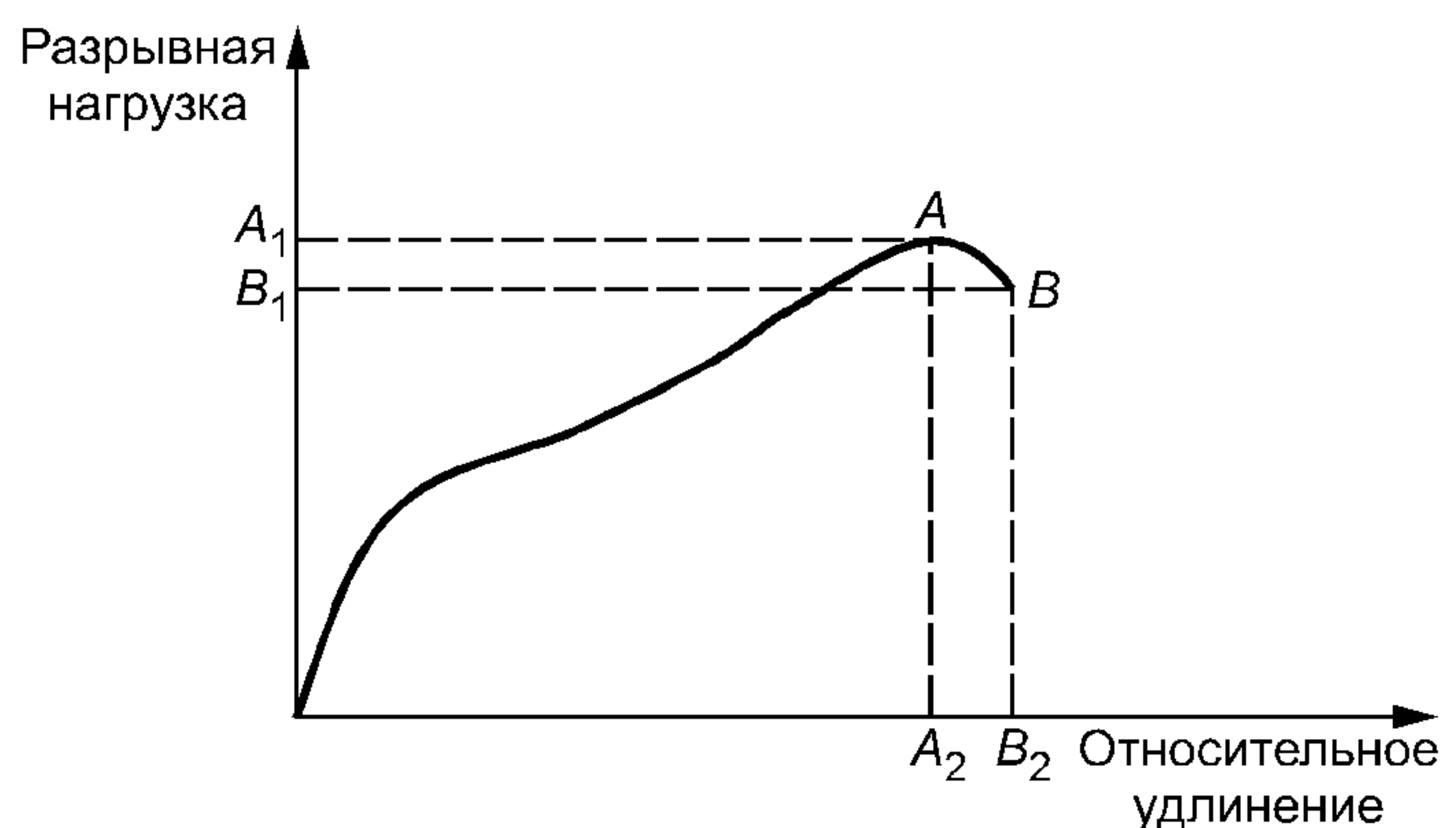
Рисунок 1 — Типичная кривая разрывная нагрузка — относительное удлинение
