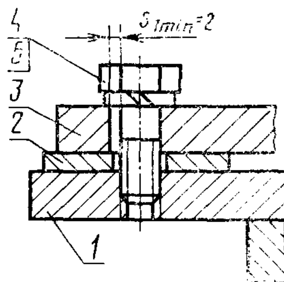
1—фундамент; 2—компенсирующий элемент; 3—механизм; 4—винт; 5—шайба
