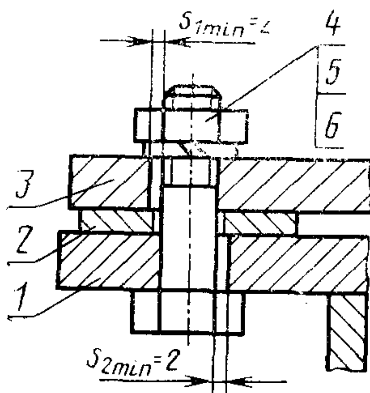
1—фундамент; 2—компенсирующий элемент; 3—механизм; 4—гайка; 5—шайба; 6—болт
