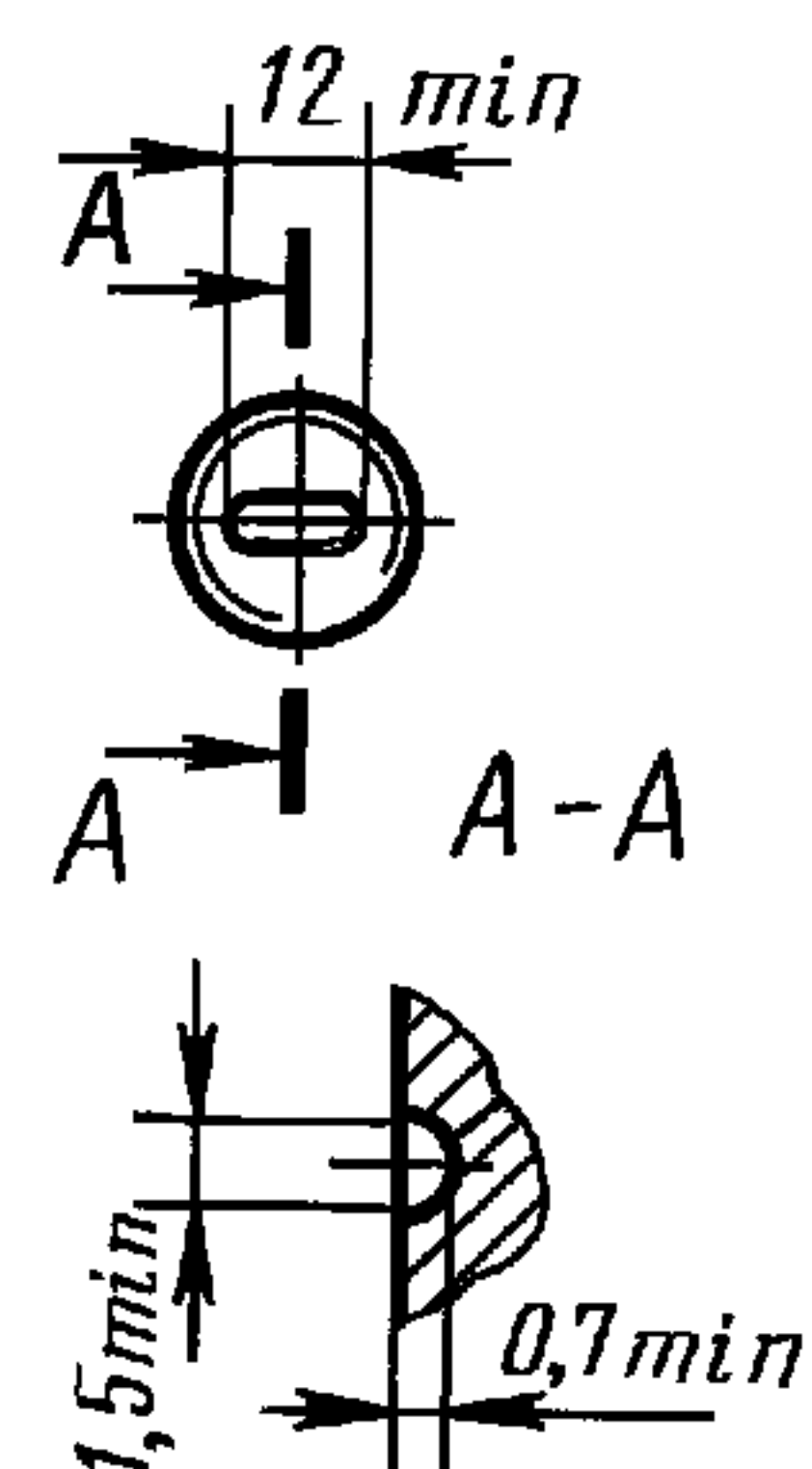
Вариант указательной канавки
