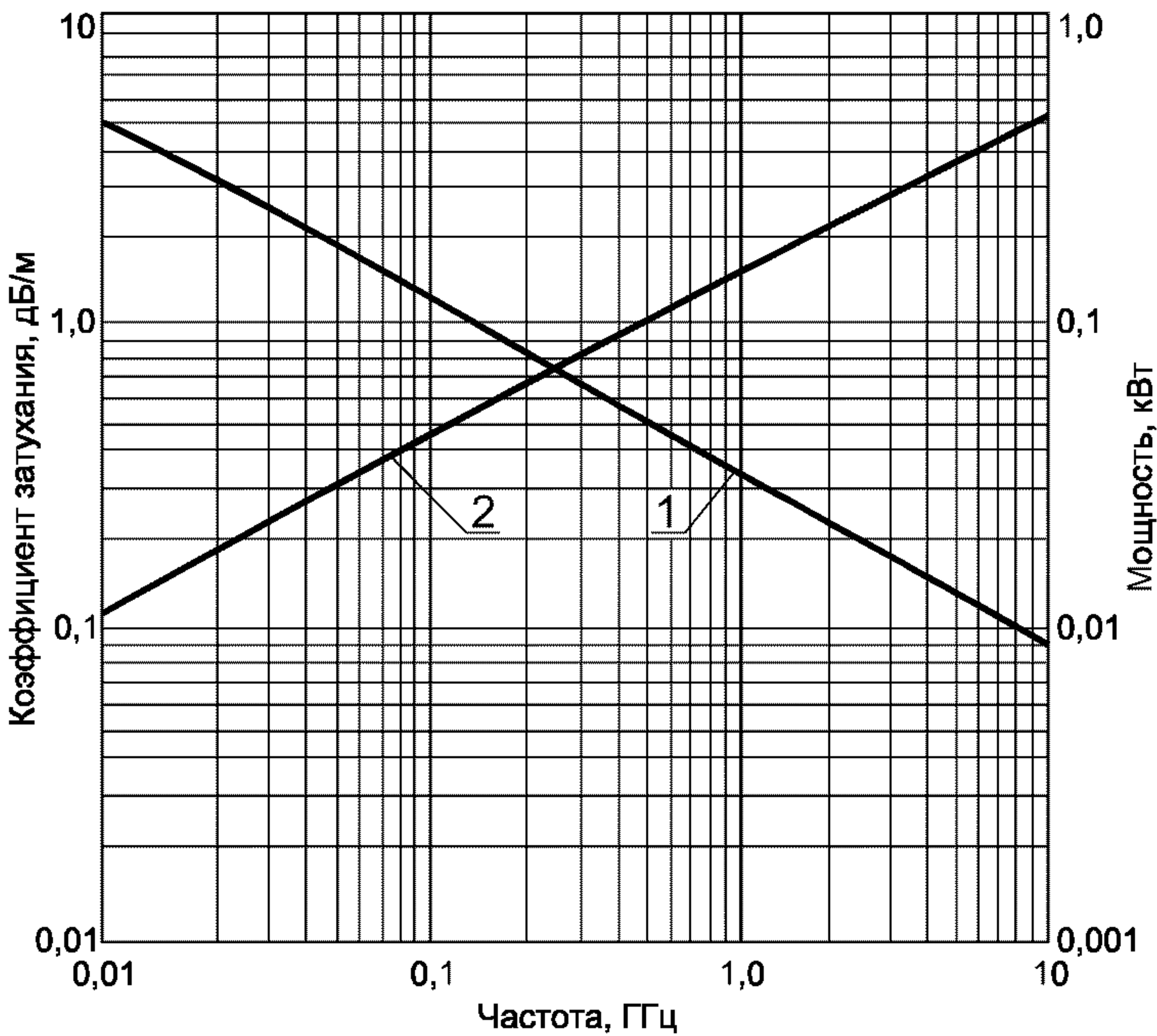
Частотные зависимости
