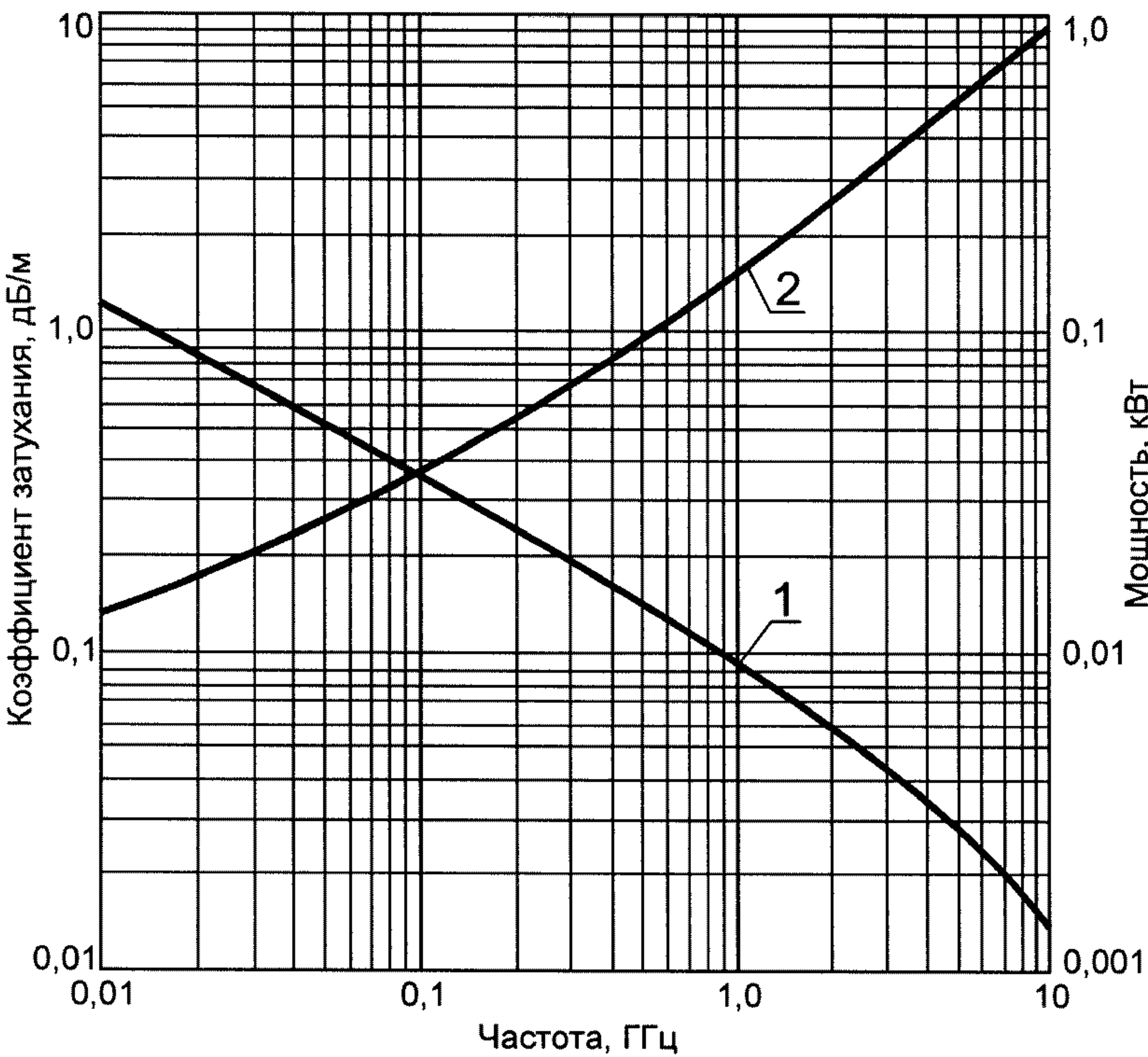
Частотные зависимости
