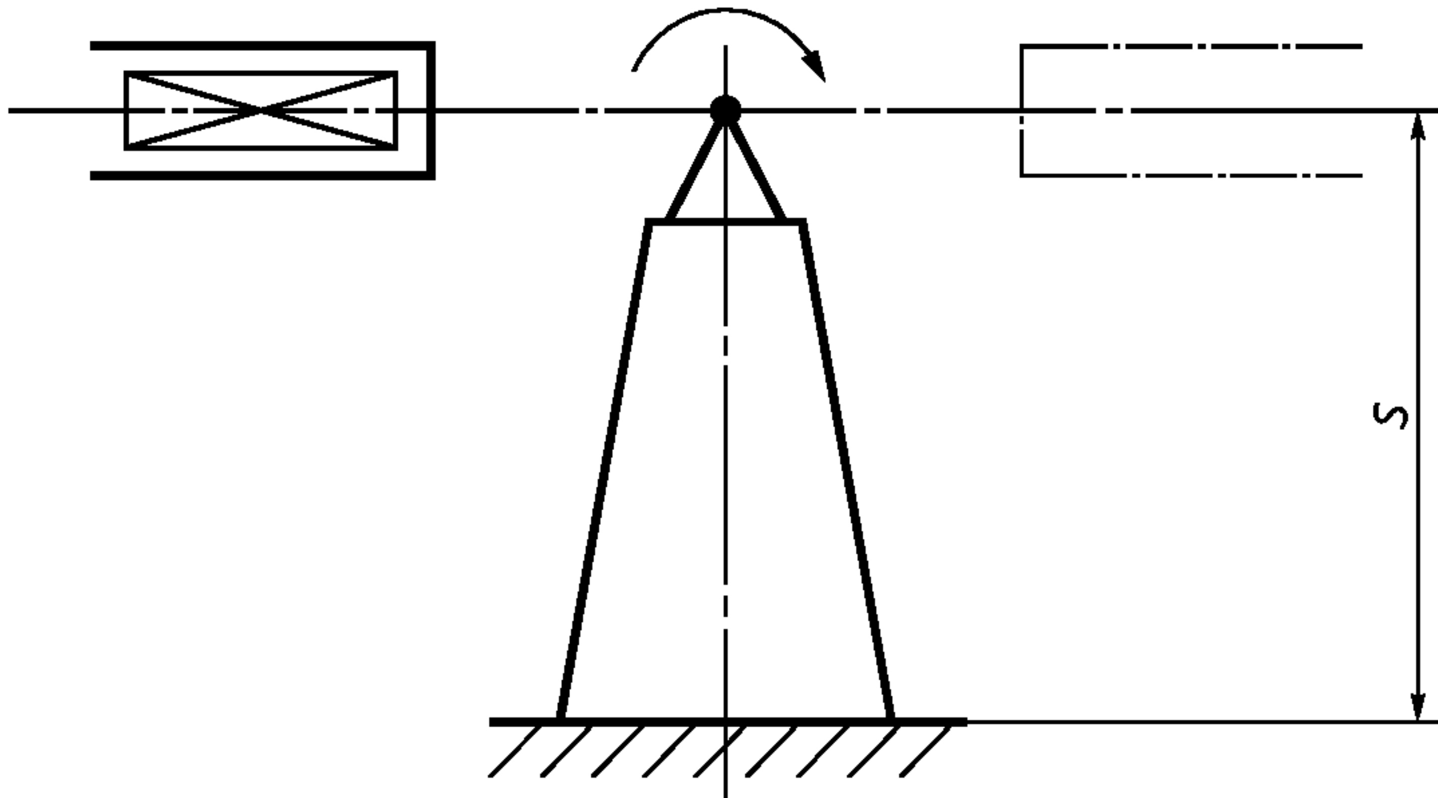
Рисунок А.9 — Кантователь рычажный (вилочный)
