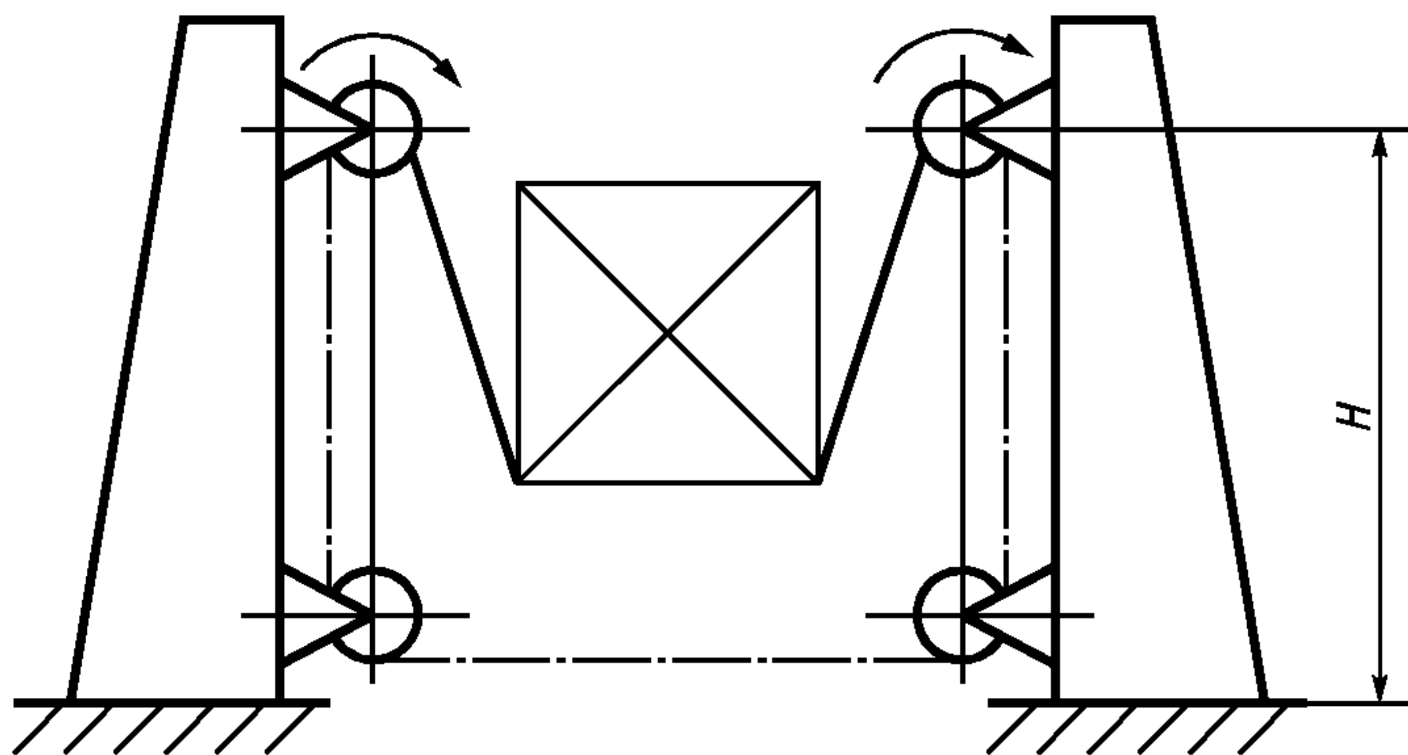
Рисунок А.12 — Кантователь цепной с четырьмя звездочками
