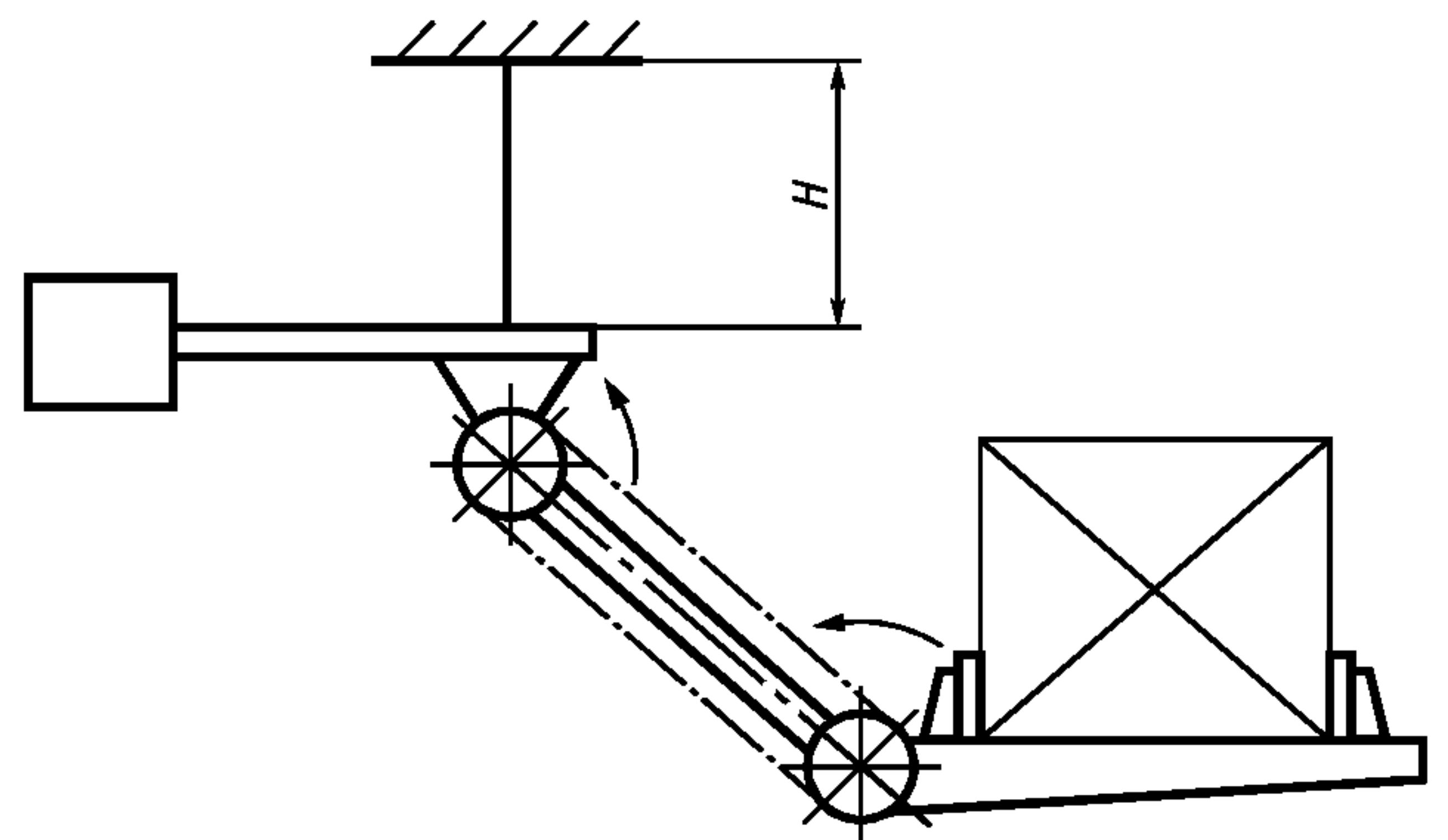
Рисунок А.16 — Кантователь рычажной подвесной
