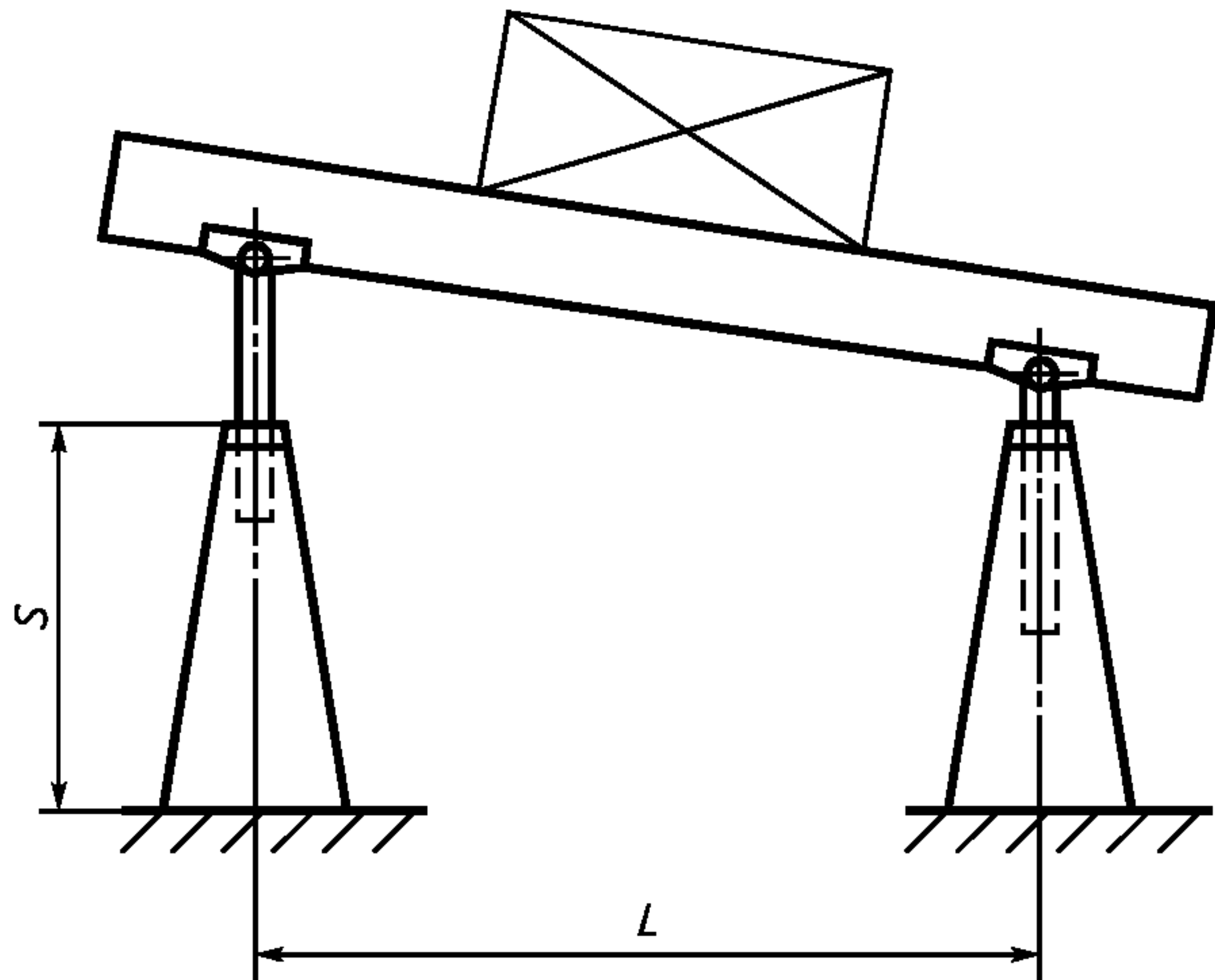
Рисунок А.8 — Кантователь рычажный двухстоечный
