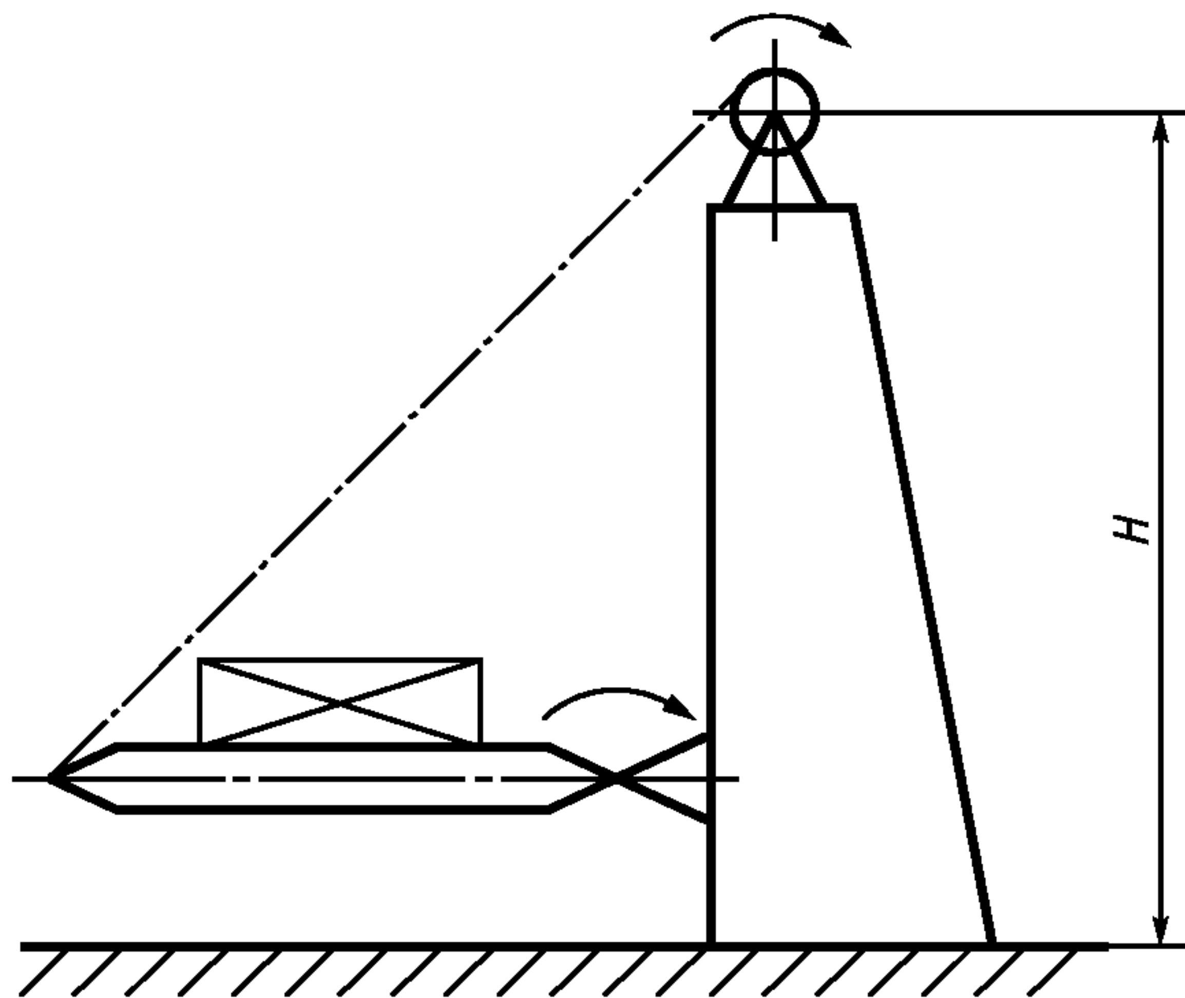
Рисунок А.10 — Кантователь рычажный с поворотной рамой
