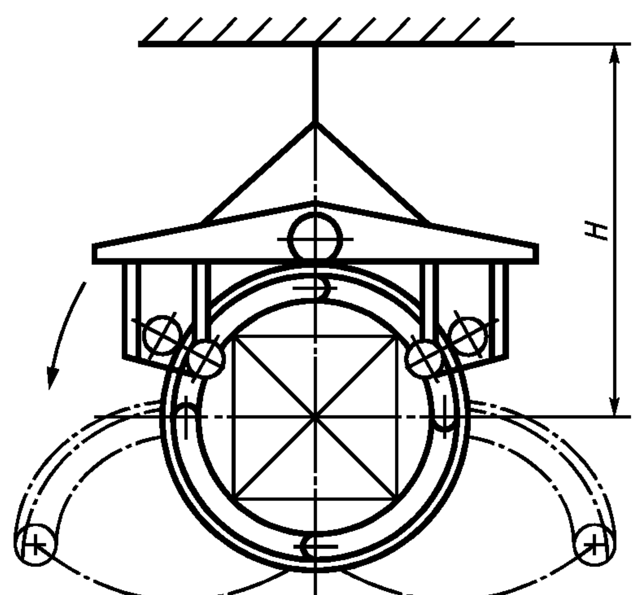
Рисунок А.18 — Кантователь центровой (кольцевой) подвесной
