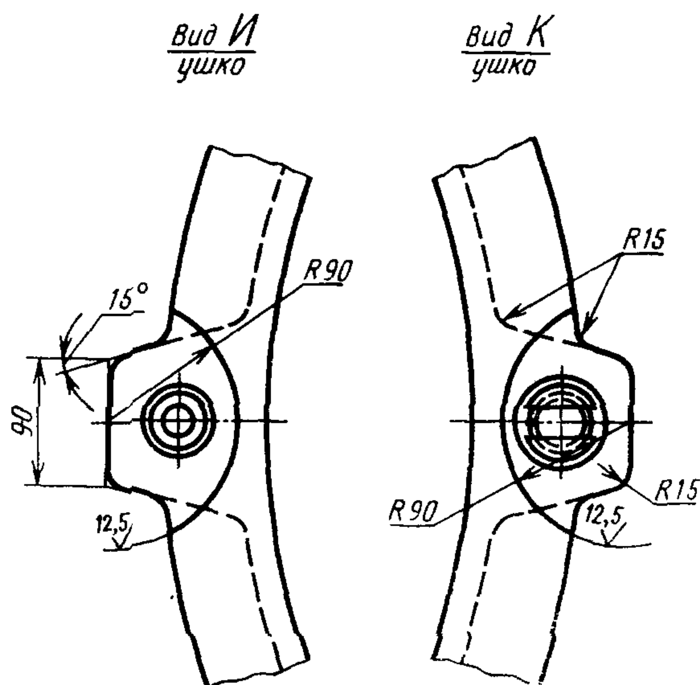
Размеры в мм
