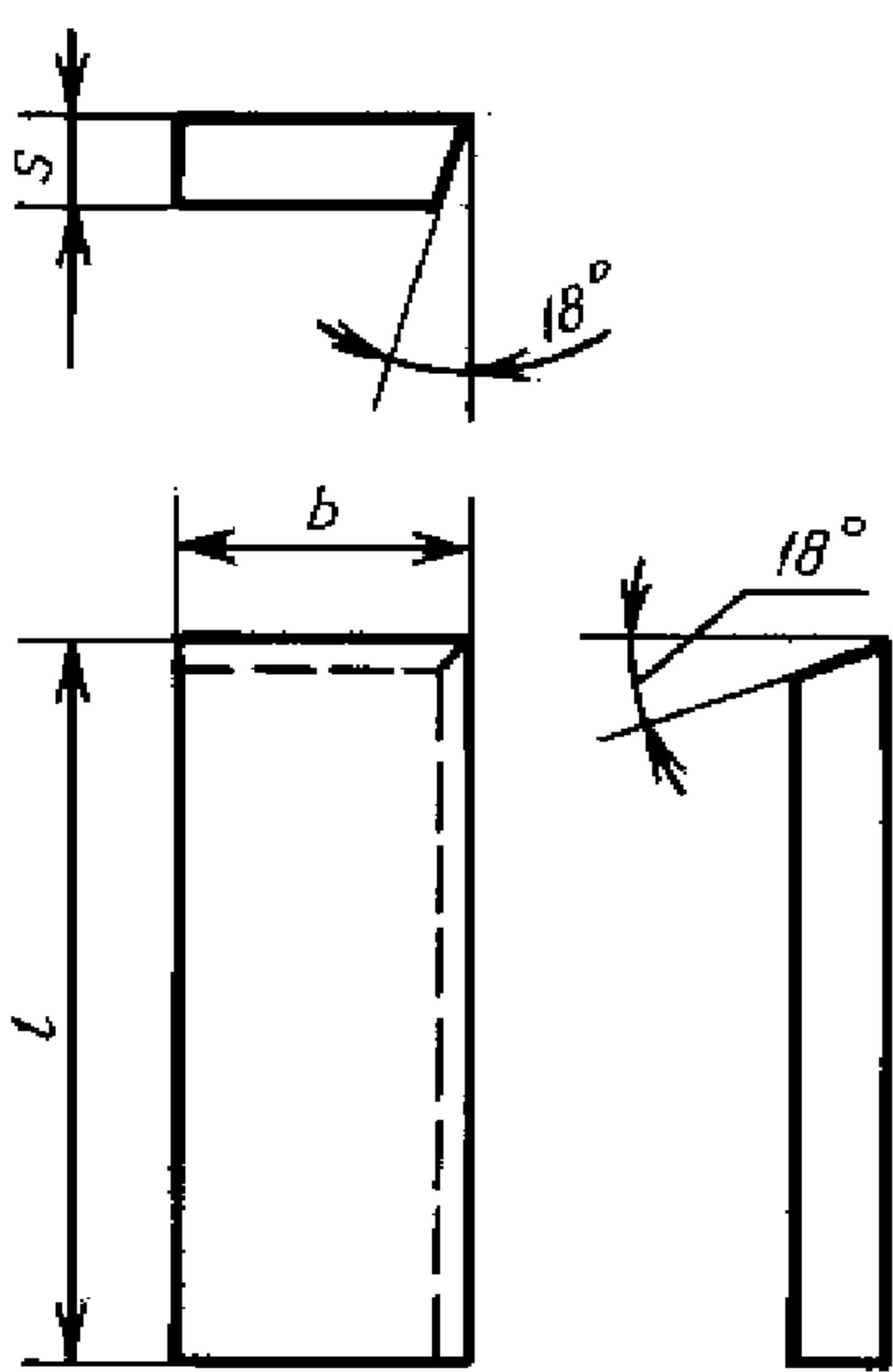
ИСПОЛНЕНИЕ 2 для обработки верхней части паза
