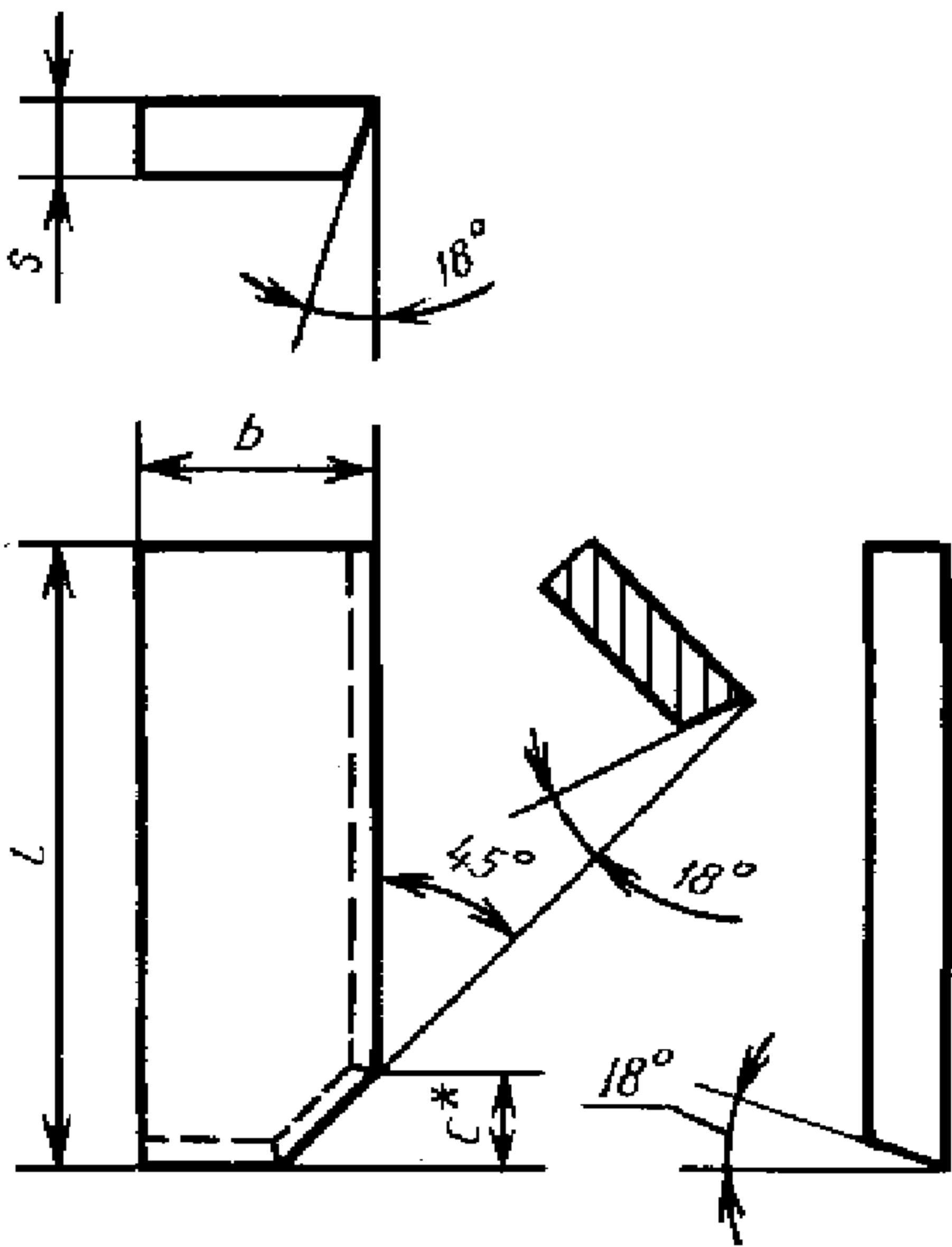
ИСПОЛНЕНИЕ 1 для обработки нижней части паза
