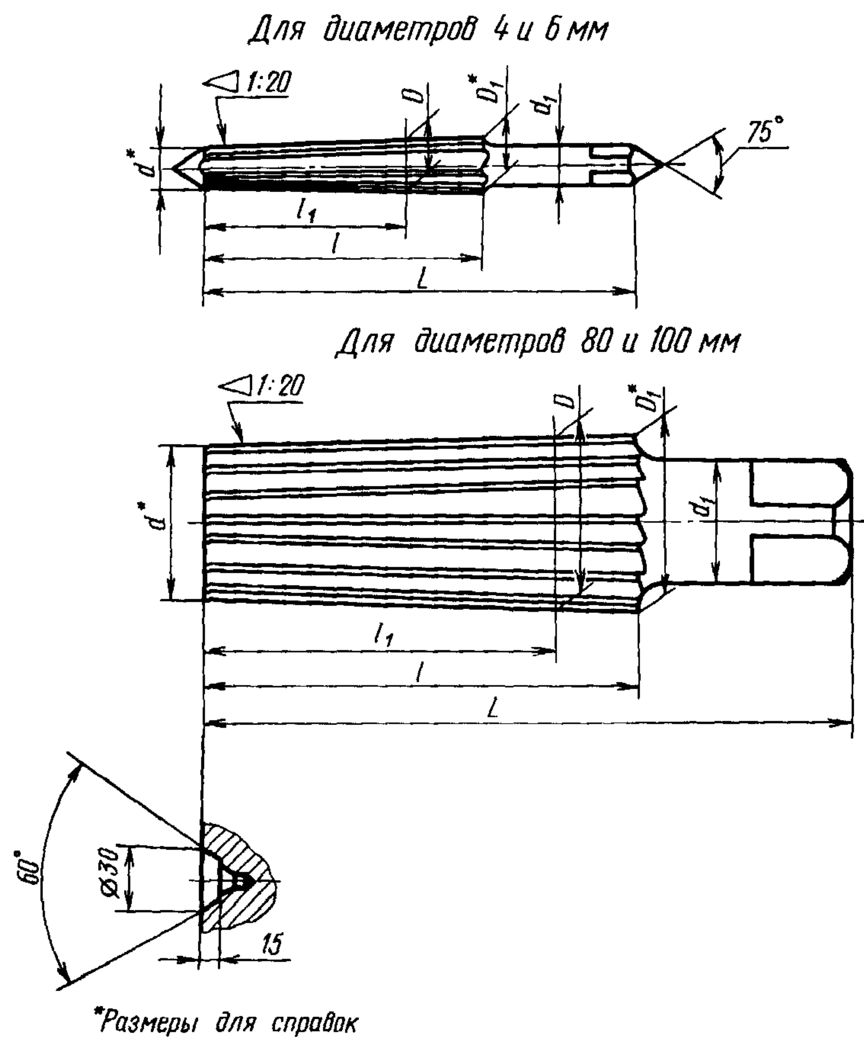
Размеры, мм
