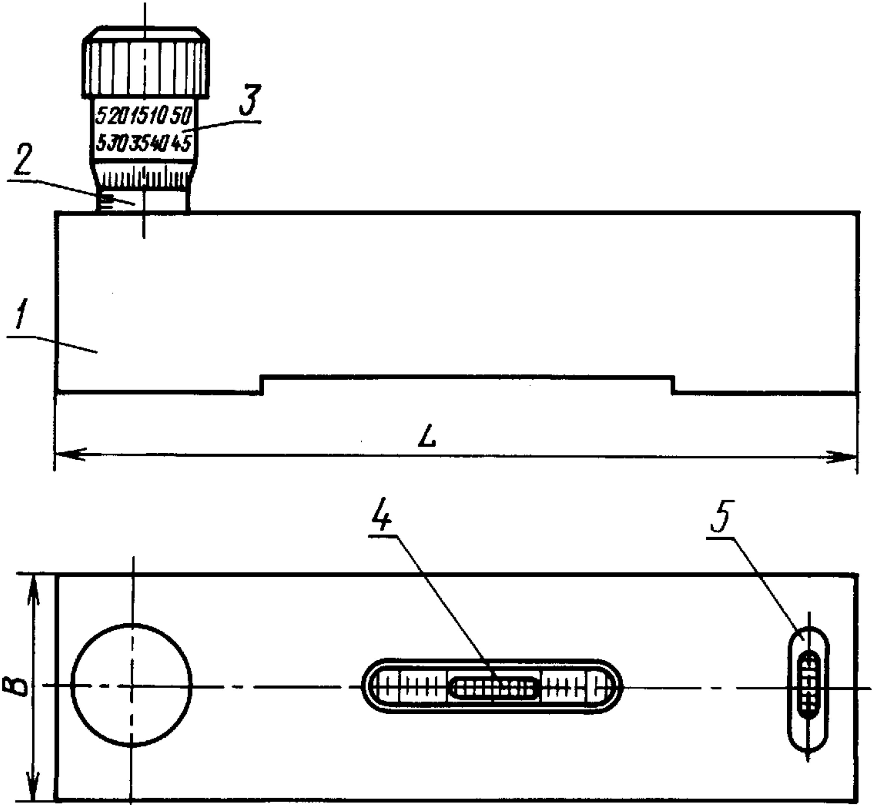
1 — основание; 2 — стебель; 3 — барабан; 4 — продольная ампула; 5 — поперечная ампула
