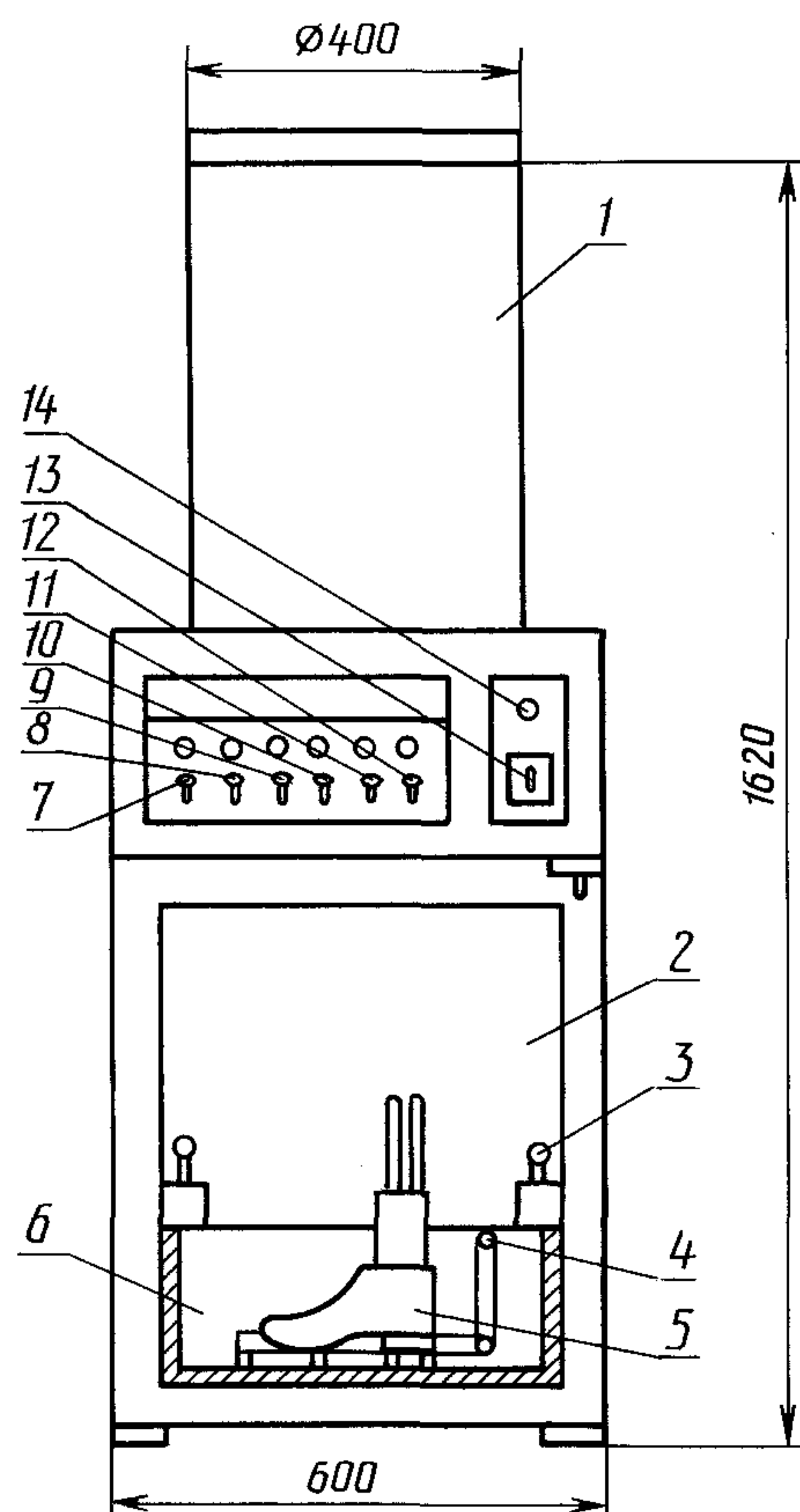
Прибор для определения пылепроницаемости спецобуви ЭПОП
