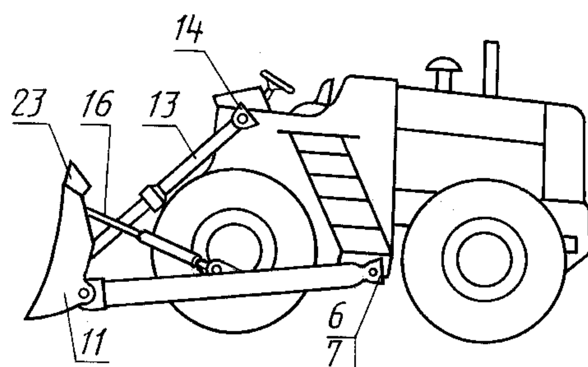
ж) Дополнительное бульдозерное оборудование
