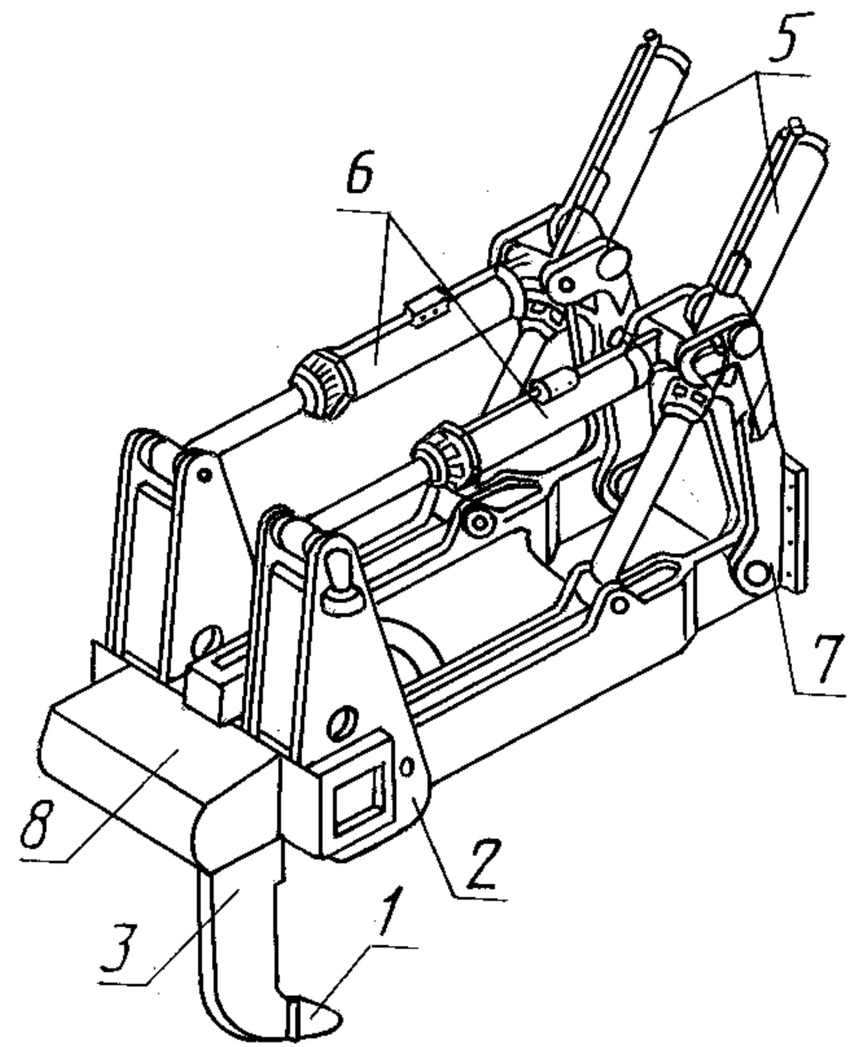
б) С регулируемым углом рыхления
