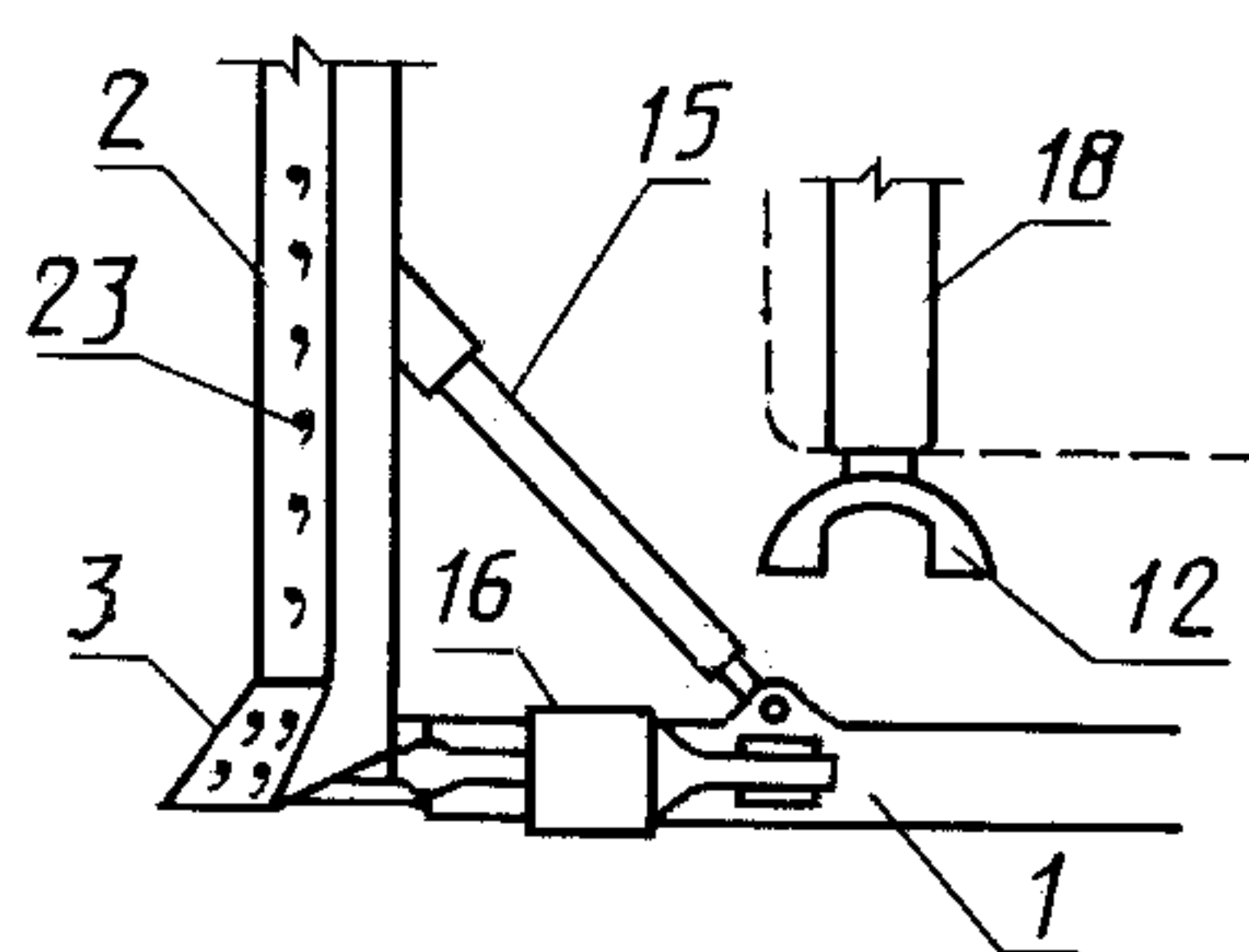
е) Отвал с амортизаторами
