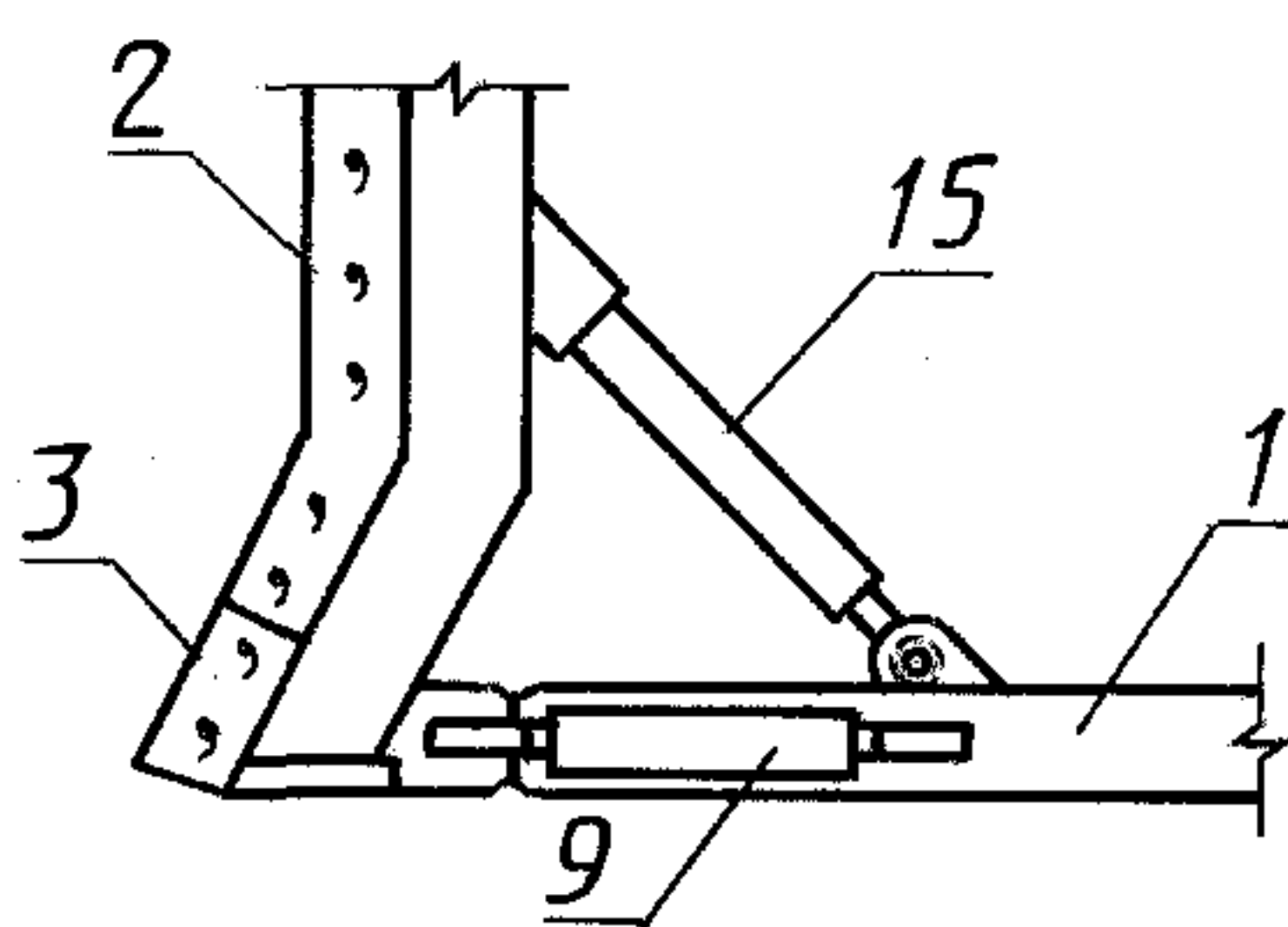
ж) Дополнительное бульдозерное оборудование
