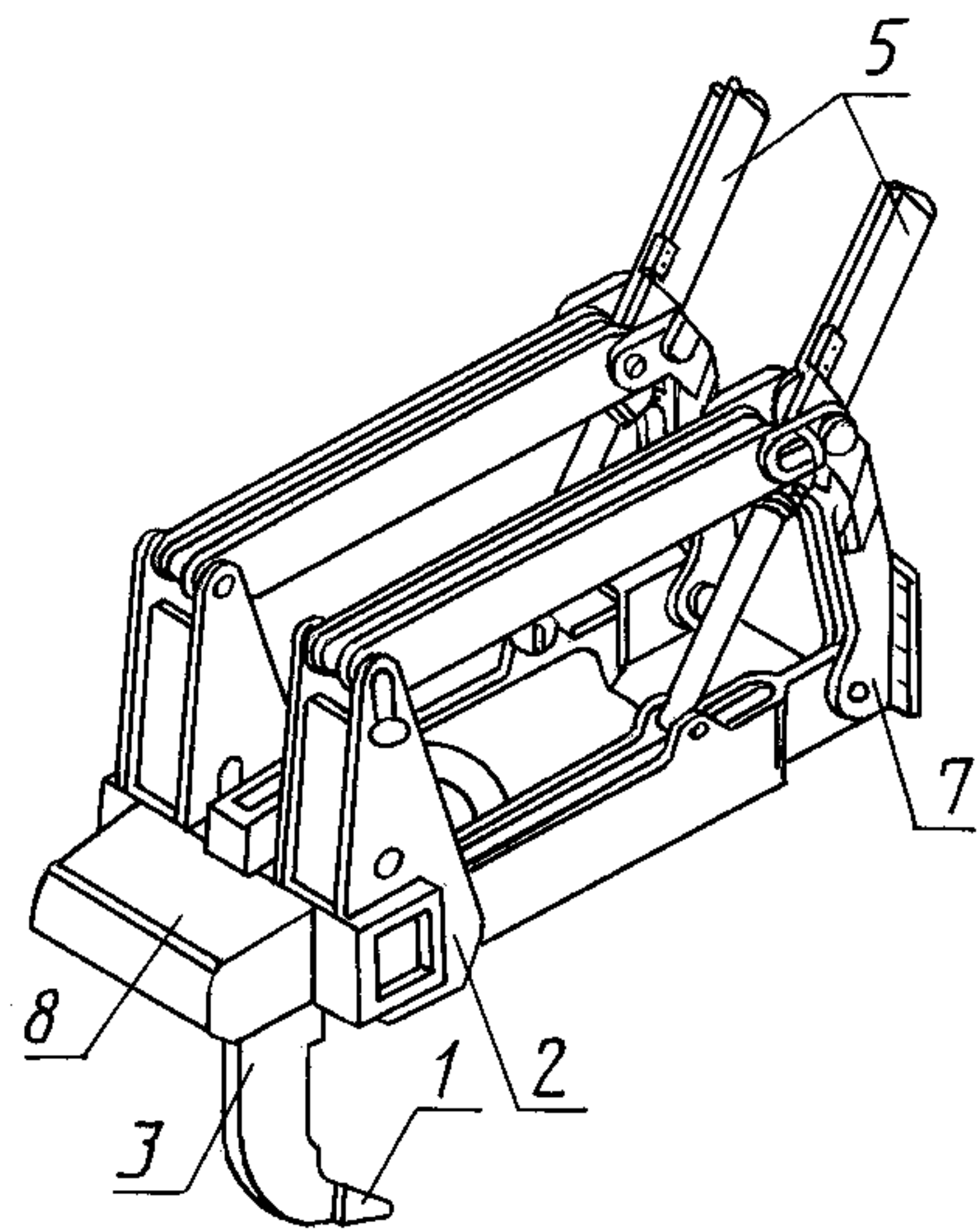
в) Трехзвенное
