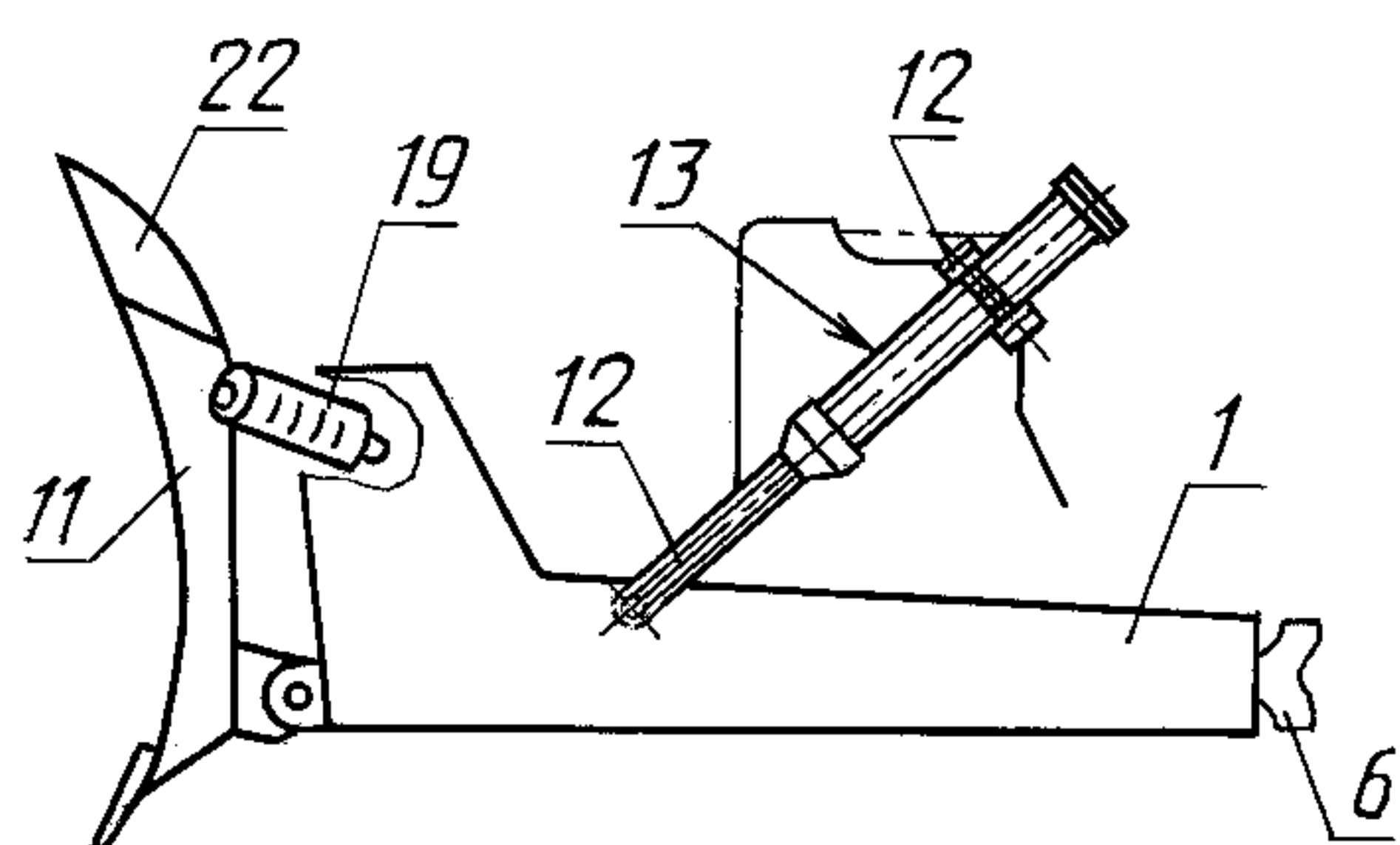
е) Отвал с амортизаторами
