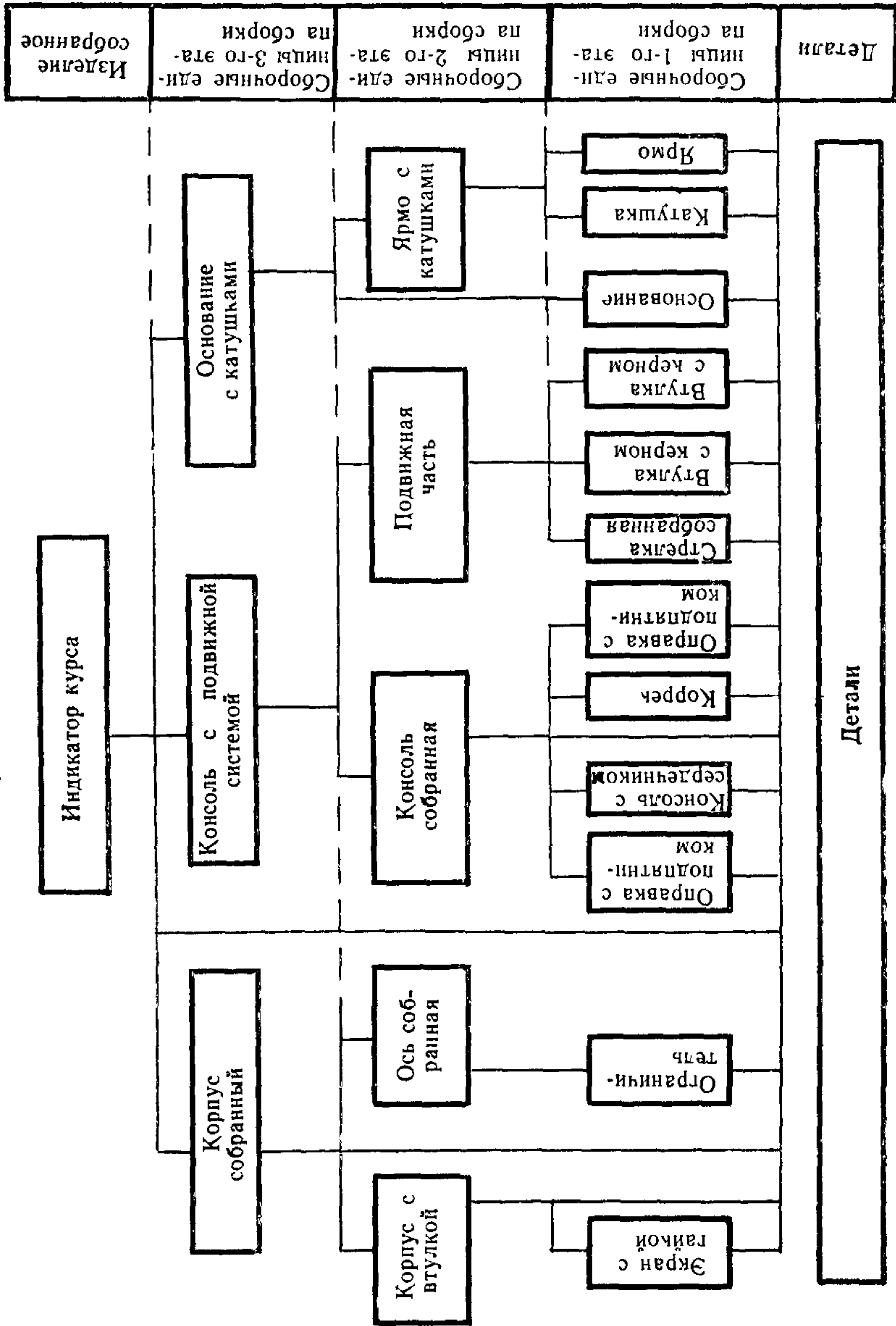
Схема сборки индикатора курса
